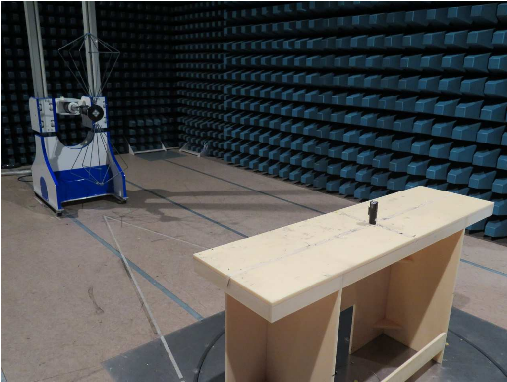
30MHz – 200MHz
