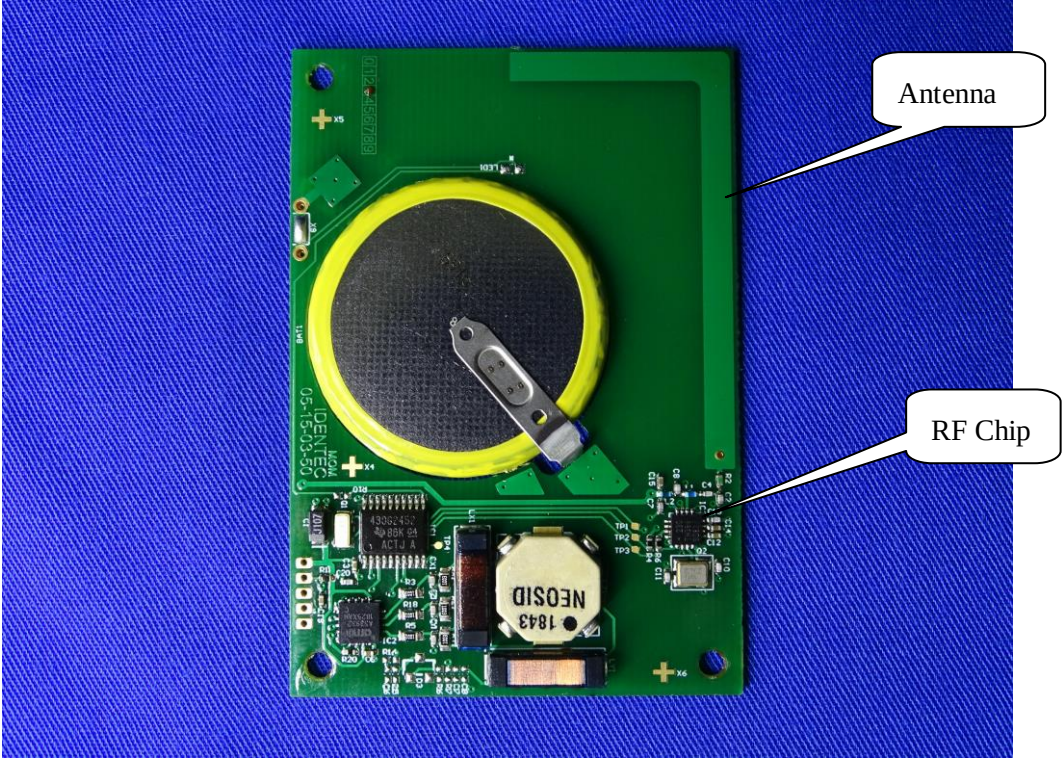
(12) EUT Photo
