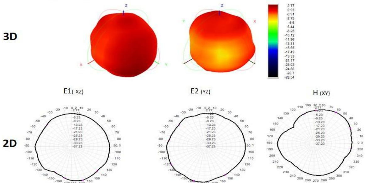
正常状态-2450MHz
