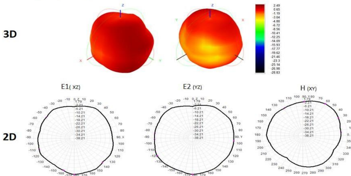
正常状态-2400MHz
