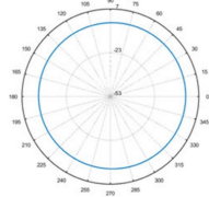
Total-Polar-H-920MHZ
