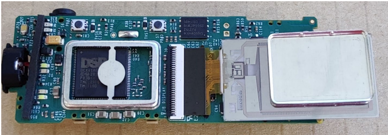
PCBA side 2 B
