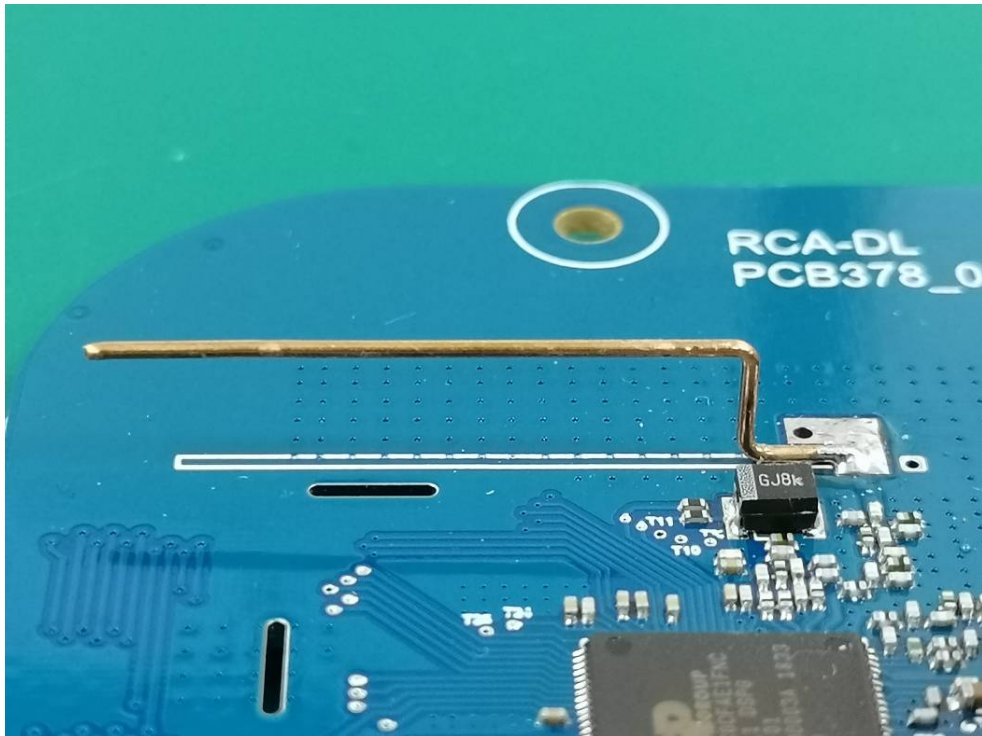
ANT1
