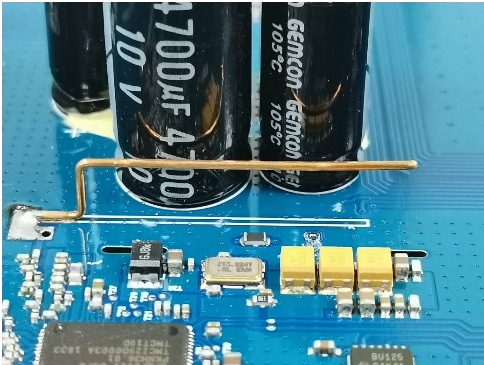
ANT0
