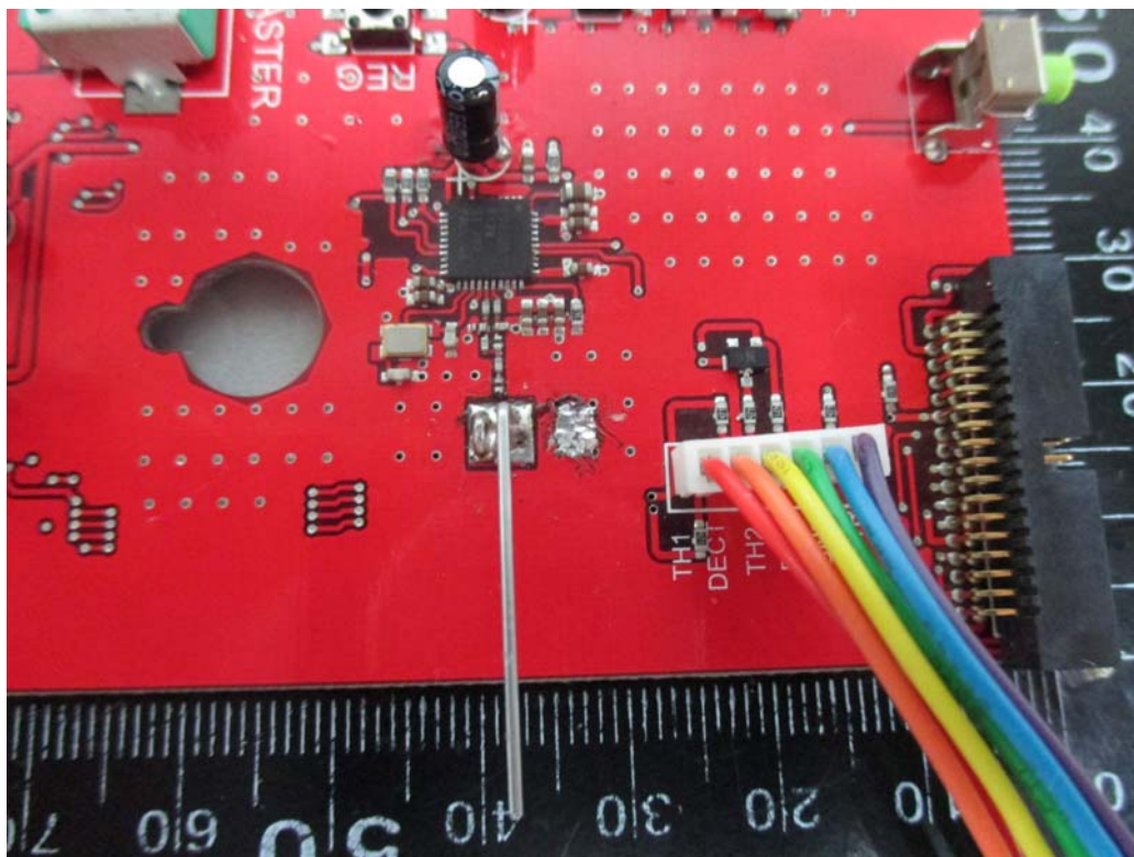
5. Zigbee Module
