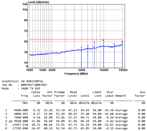
Headset 2.4G SRD_2M_TX_CH_39_Horizontal-Avg
