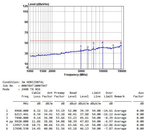
Headset 2.4G SRD_1M_TX_CH_39_Horizontal-Avg
