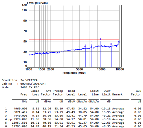
Headset 2.4G SRD_2M_TX_CH_39_Vertical-Avg
