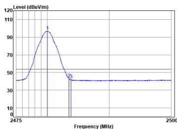
Headset 2.4G SRD_2M_TX_CH_39_Horizontal-Avg
