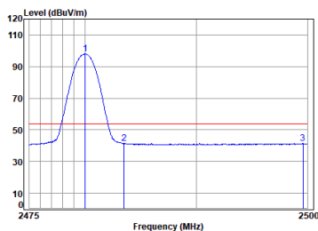
Headset 2.4G SRD_1M_TX_CH_39_Horizontal-Avg
