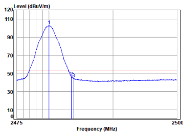
Headset 2.4G SRD_TX_CH_39_Vertical-Avg
