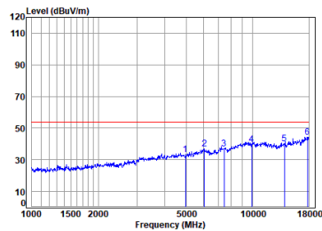
Headset BLE_2M_TX_CH_39_Vertical-Avg
