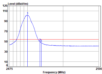
Headset BLE_2M_TX_CH_39_Horizontal-Avg
