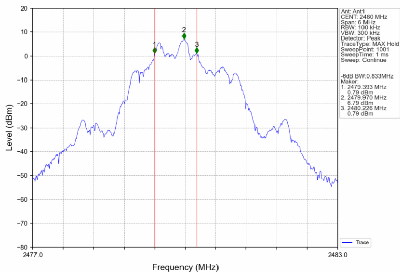
2M_HCH_2480MHz_Ant1_NTNV
