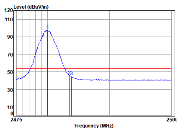
Headset BLE_2M_TX_CH_39_Vertical-Avg
