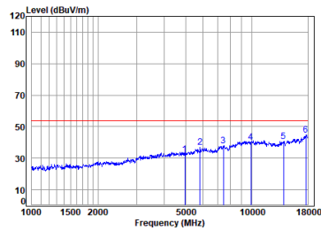
Headset BLE_2M_TX_CH_39_Horizontal-Avg
