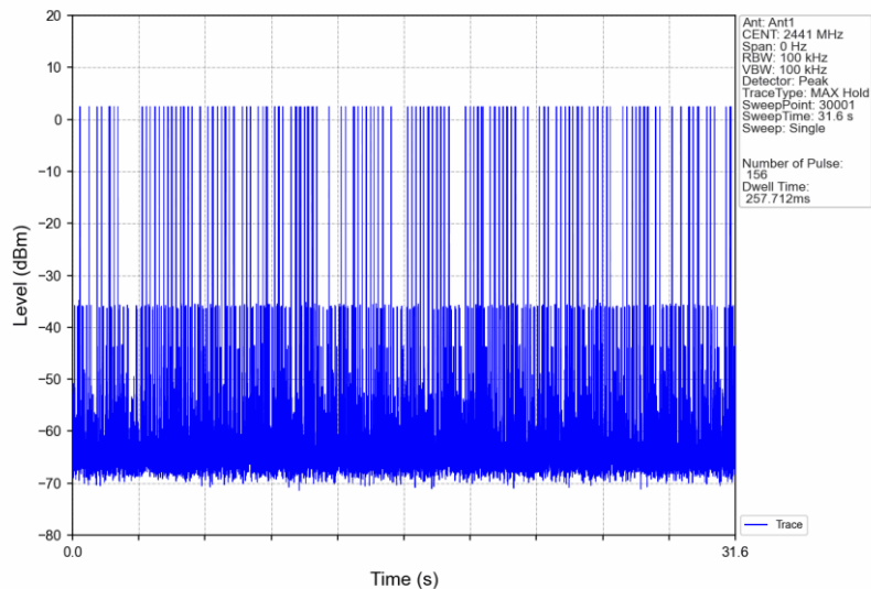
GFSK_DH3_HOPP_Ant1_NTNV
