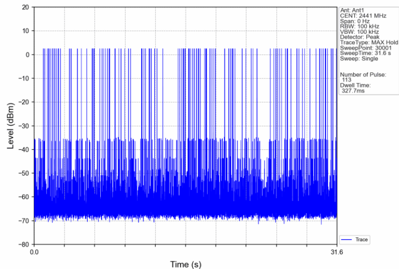
GFSK_DH5_HOPP_Ant1_NTNV
