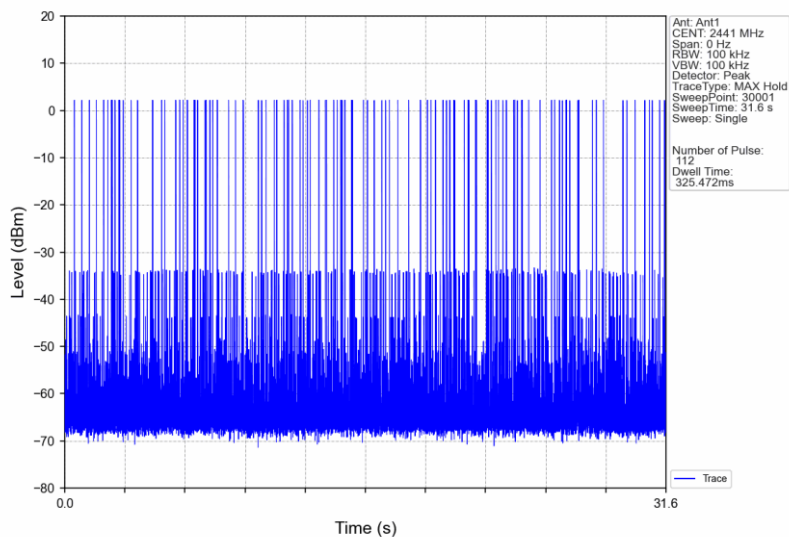
Pi/4DQPSK_2DH5_HOPP_Ant1_NTNV
