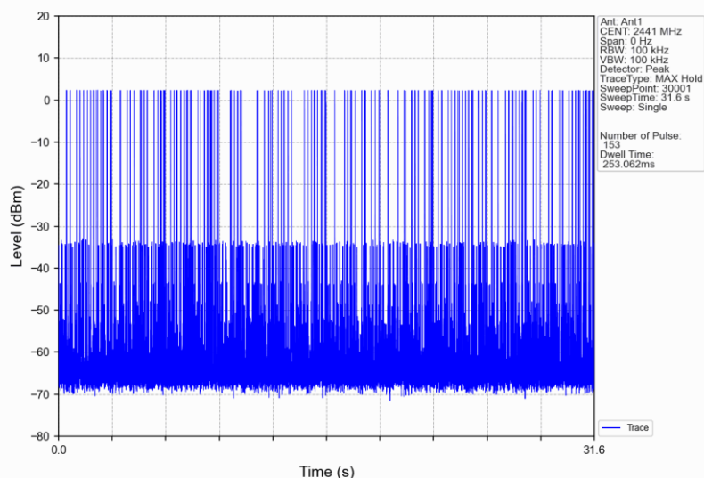
Pi/4DQPSK_2DH3_HOPP_Ant1_NTNV
