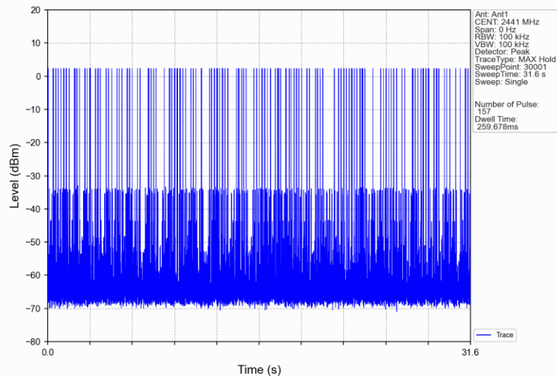
8DPSK_3DH3_HOPP_Ant1_NTNV
