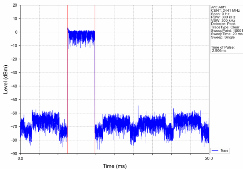
Pi/4DQPSK_2DH5_HOPP_Ant1_NTNV
