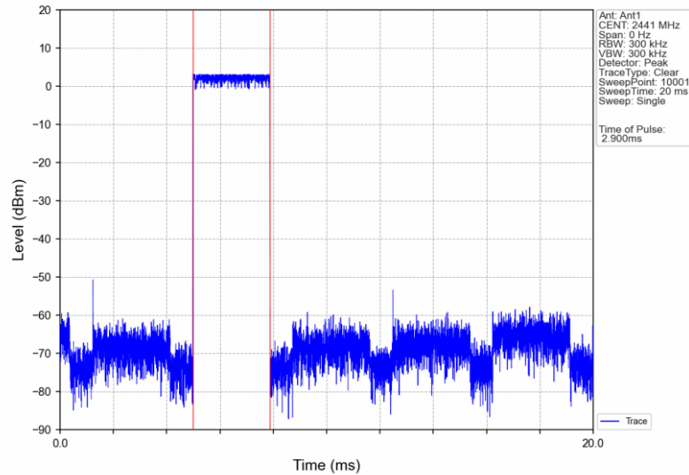
GFSK_DH5_HOPP_Ant1_NTNV
