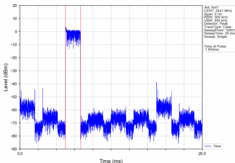
Pi/4DQPSK_2DH3_HOPP_Ant1_NTNV
