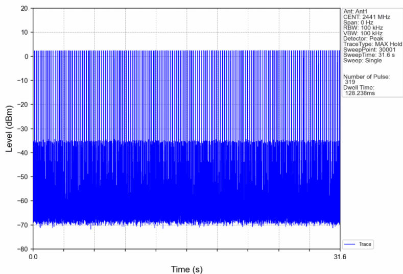
Pi/4DQPSK_2DH1_HOPP_Ant1_NTNV
