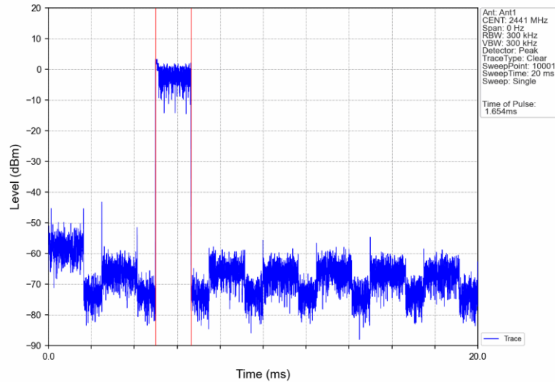
8DPSK_3DH3_HOPP_Ant1_NTNV
