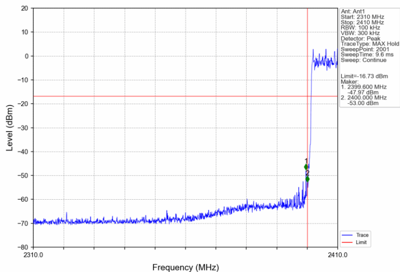
Pi/4DQPSK_2DH5_HOPP_Ant1_NTNV
