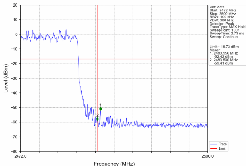
Pi/4DQPSK_2DH5_HOPP_Ant1_NTNV
