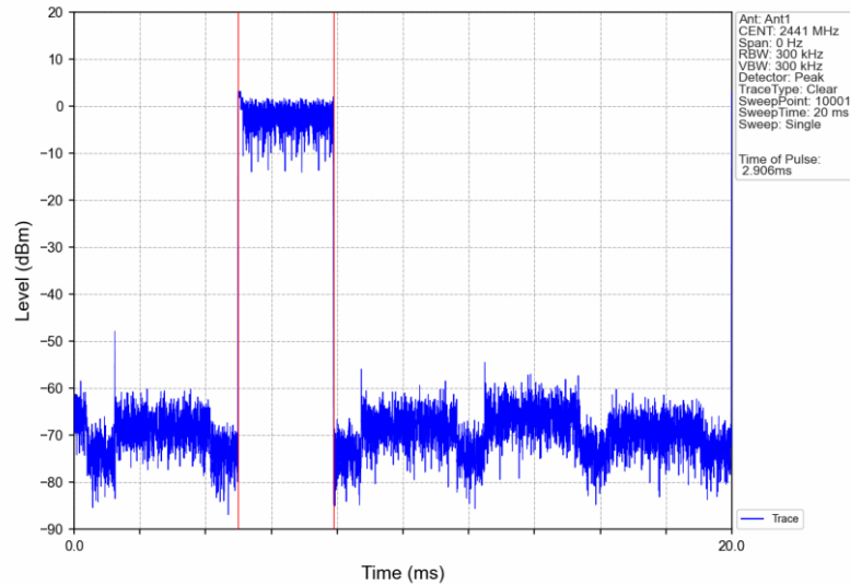
8DPSK_3DH5_HOPP_Ant1_NTNV
