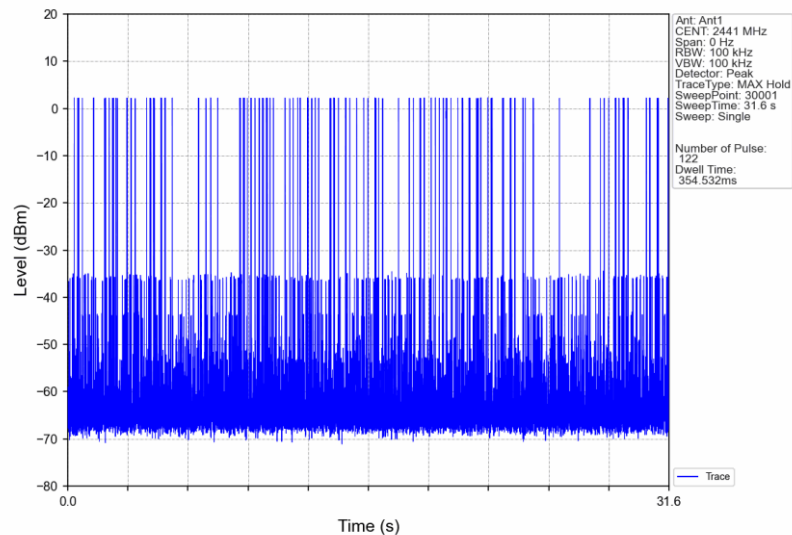
8DPSK_3DH5_HOPP_Ant1_NTNV
