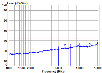
Dongle 2.4SRD_1M_TX_CH_39_Vertical-Avg
