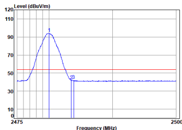
Dongle 2.4G SRD_2M_TX_CH_39_Horizontal-Avg
