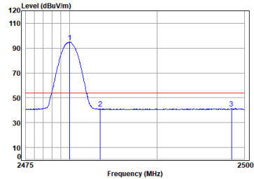
Dongle 2.4G SRD_1M_TX_CH_39_Horizontal-Avg
