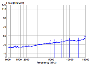
Dongle 2.4SRD_1M_TX_CH_39_Horizontal-Avg
