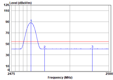
Dongle 2.4G SRD_1M_TX_CH_39_Vertical-Avg
