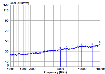
Dongle 2.4SRD_2M_TX_CH_39_Horizontal-Avg
