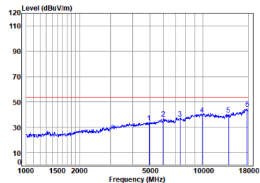
Dongle 2.4SRD_2M_TX_CH_39_Vertical-Avg
