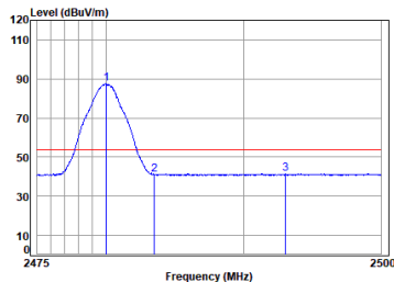
Dongle 2.4G SRD_2M_TX_CH_39_Vertical-Avg
