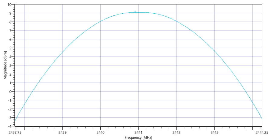
Plot_Common2G4 Peak OP 3MHz-3MHz ~ BT Classic EDR Pi-4DQPSK_09122020_151324.png
