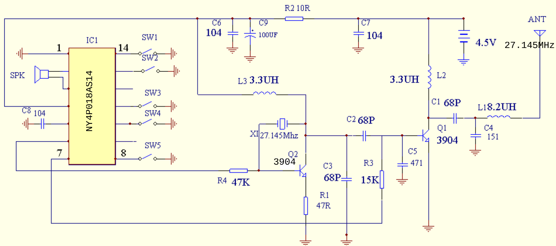
27MHz发射原理图
