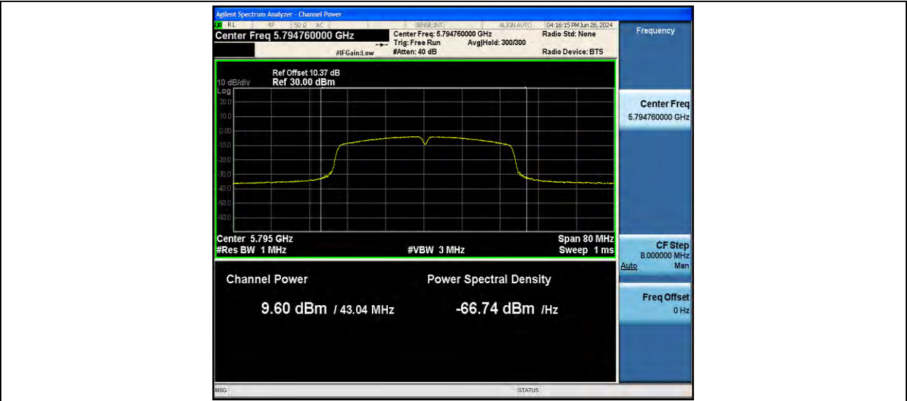
11N40SISO_Ant2_5795
