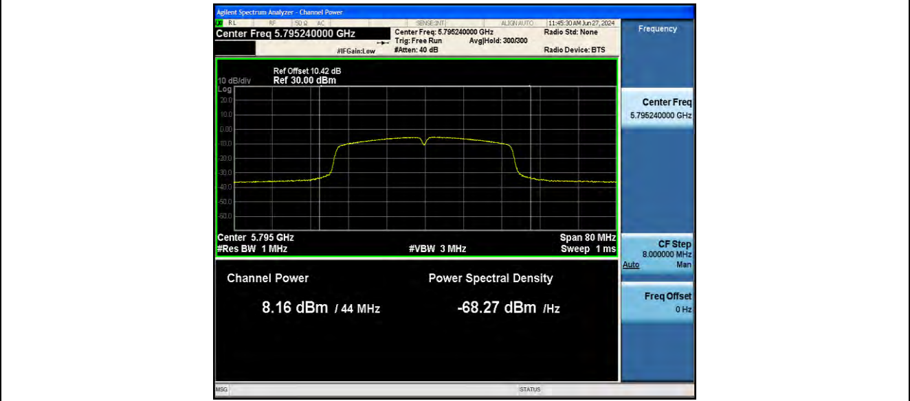
11N40SISO_Ant2_5795
