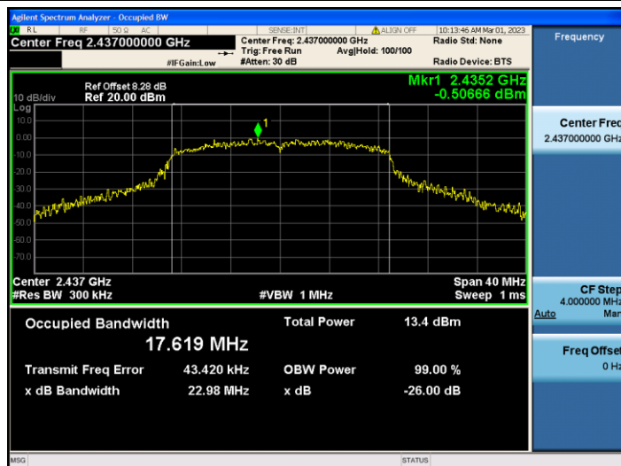
11N20MIMO_Ant2_2437
