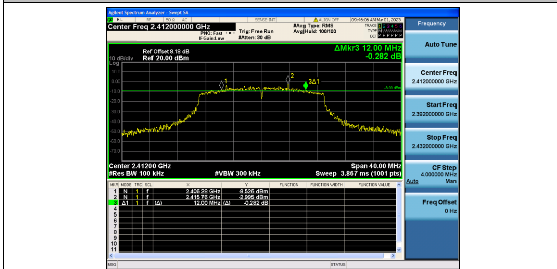
11N20MIMO_Ant2_2412
