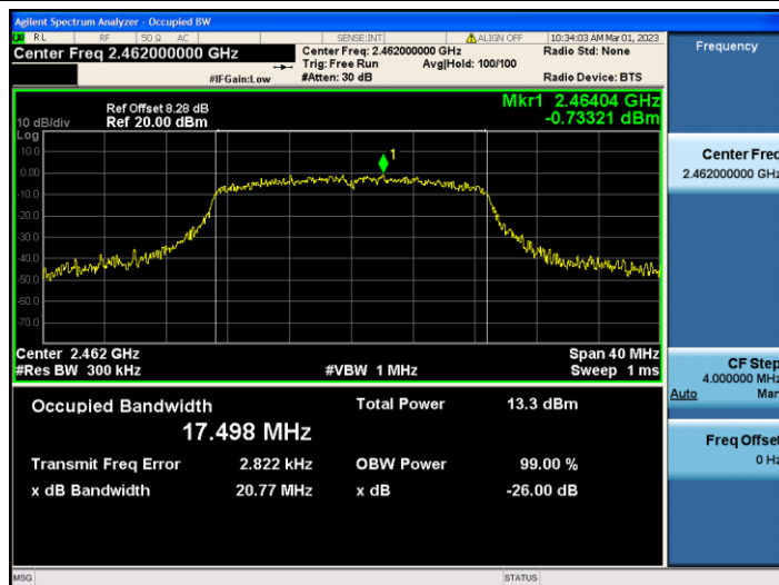
11N20MIMO_Ant2_2462
