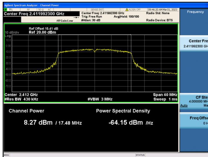
11N20MIMO_Ant2_2412
