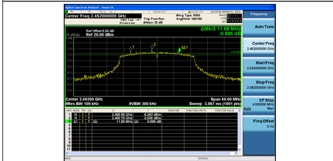
11N20MIMO_Ant2_2462
