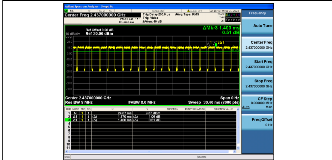
11N20MIMO_Ant2_2437
