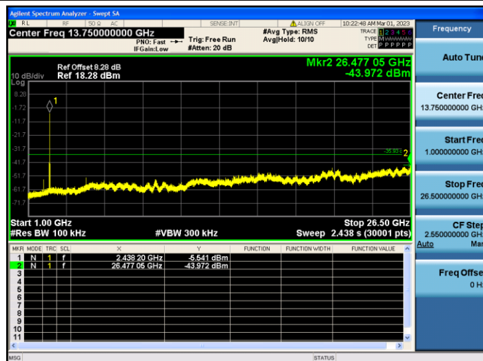
11N20MIMO_Ant2_2437_0~Reference
