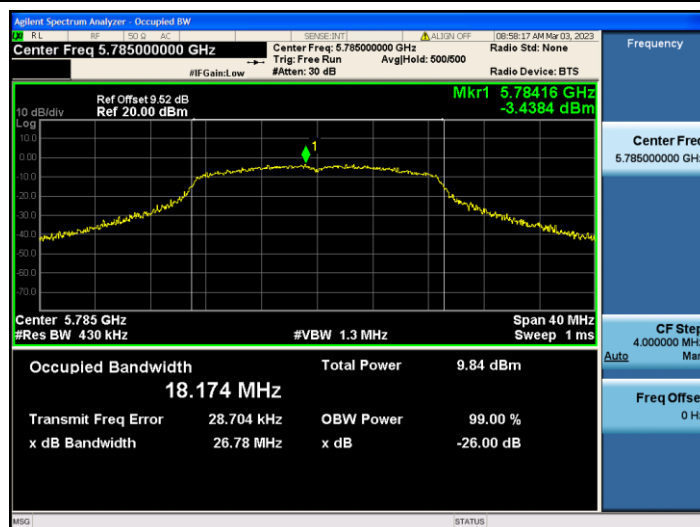
11N20SISO_Ant2_5785
