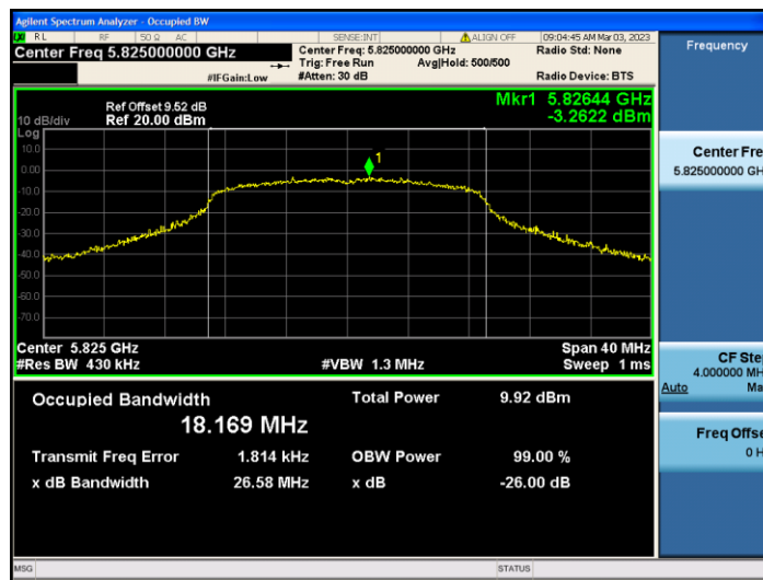
11N20SISO_Ant2_5825
