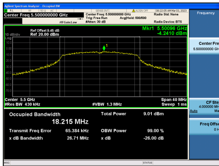
11N20SISO_Ant2_5500
