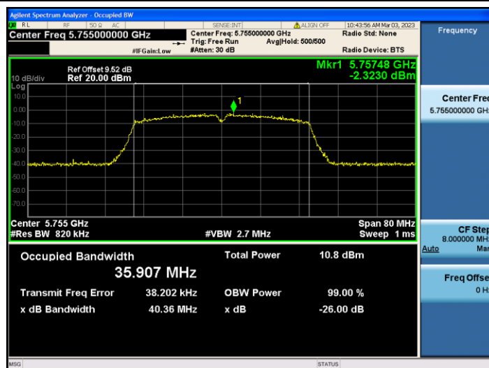
11N40SISO_Ant2_5755
