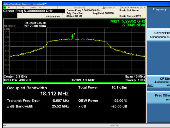
11N20SISO_Ant2_5300
