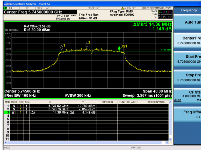
11A_Ant2_5745
