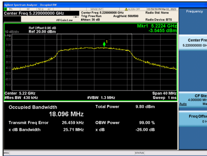
11N20SISO_Ant2_5220
