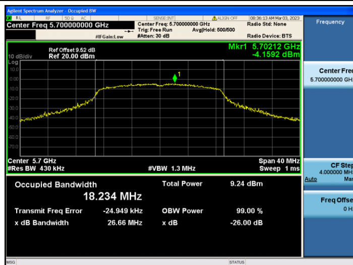
11N20SISO_Ant2_5700
