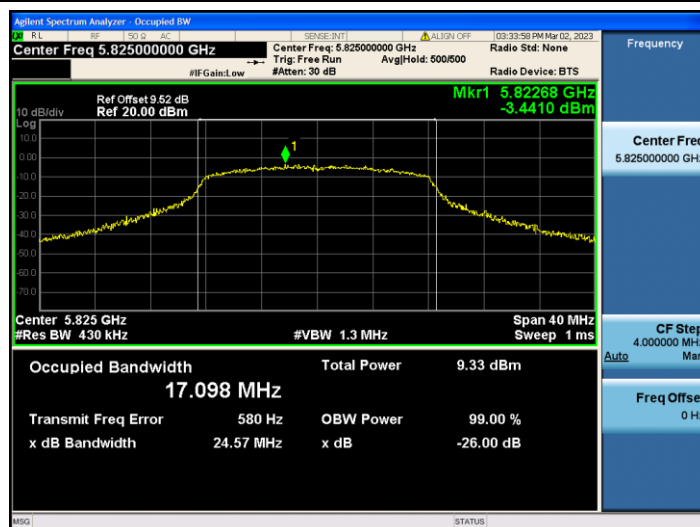
11A_Ant2_5825
