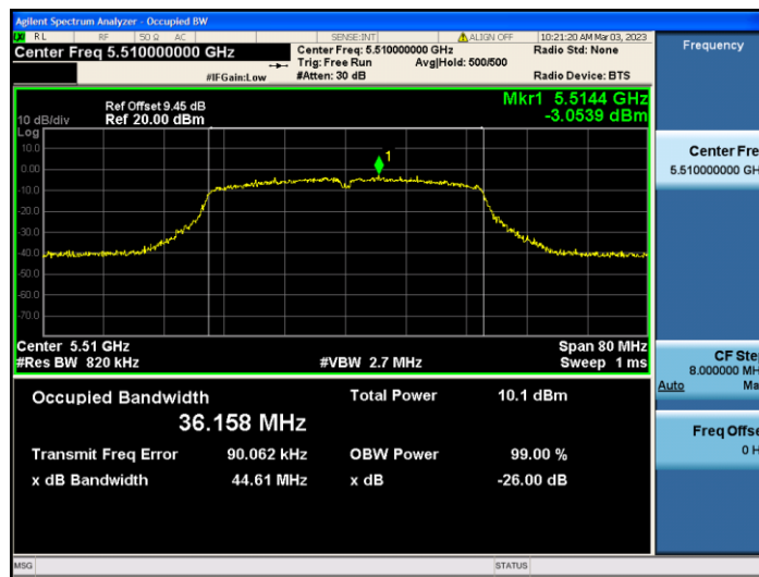
11N40SISO_Ant2_5510
