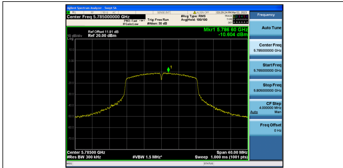
11A_Ant2_5785
