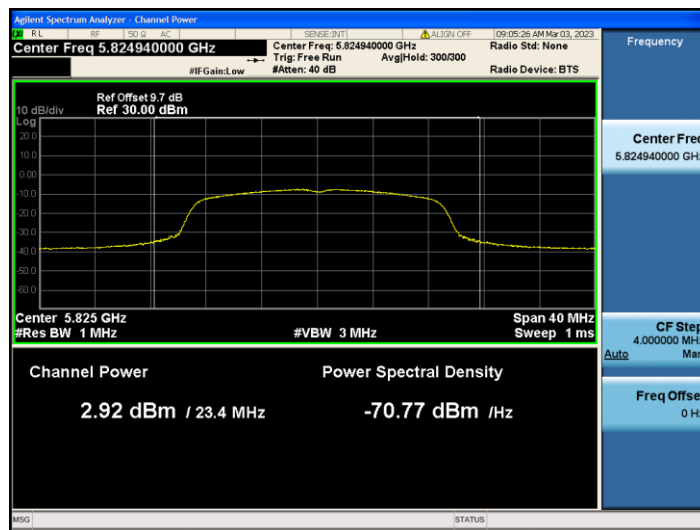
11N20SISO_Ant2_5825
