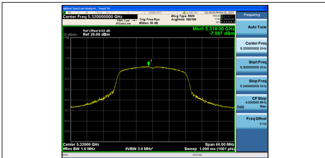
11A_Ant2_5320
