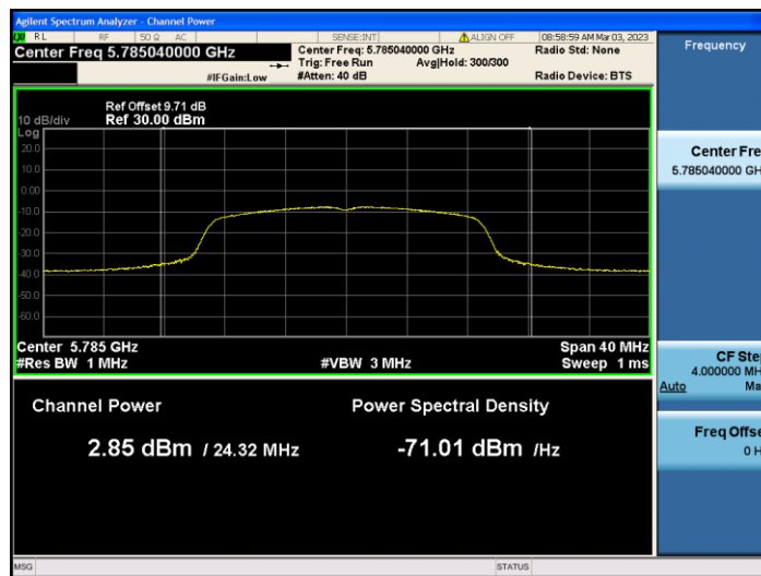
11N20SISO_Ant2_5785
