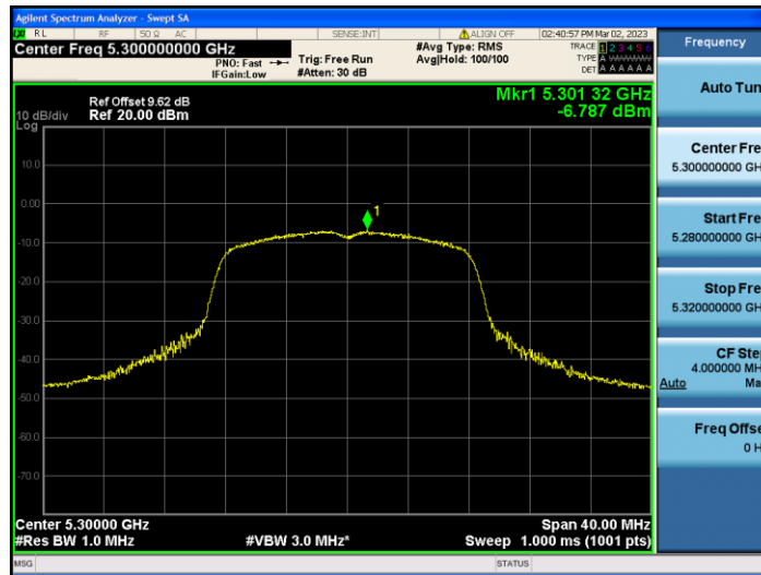
11A_Ant2_5300
