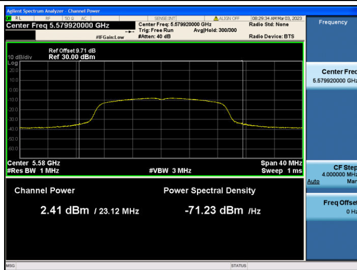
11N20SISO_Ant2_5580
