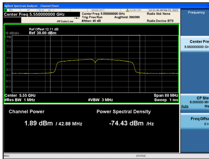
11N40SISO_Ant2_5550
