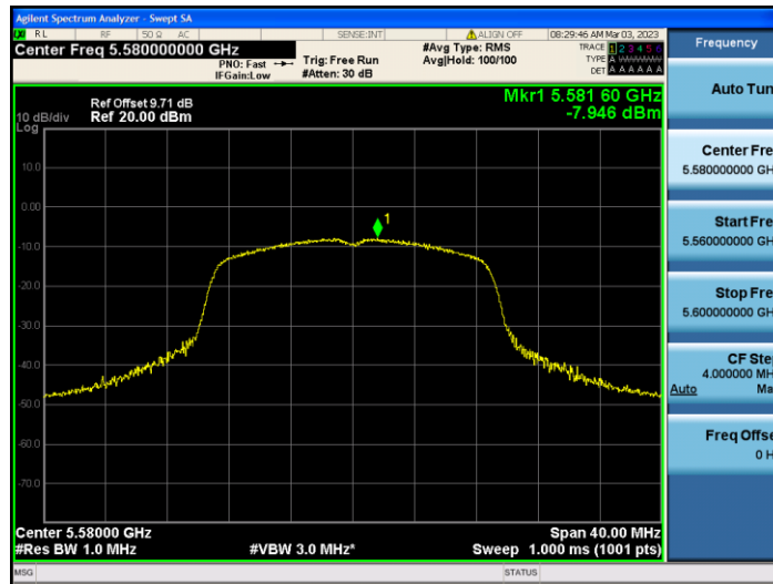
11N20SISO_Ant2_5580
