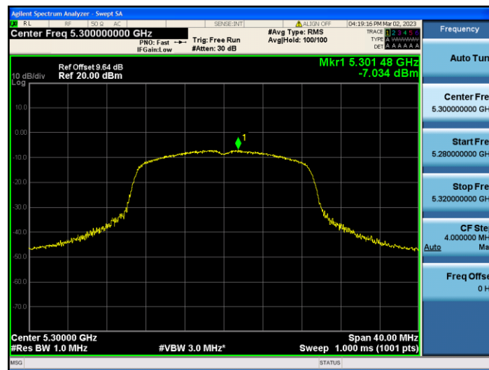
11N20SISO_Ant2_5300
