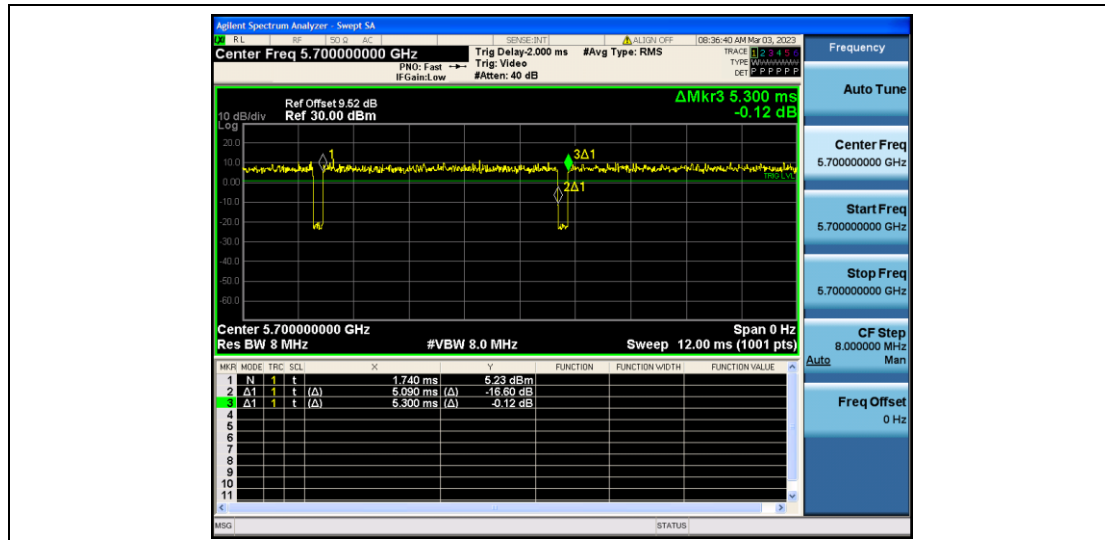
11N20SISO_Ant2_5700
