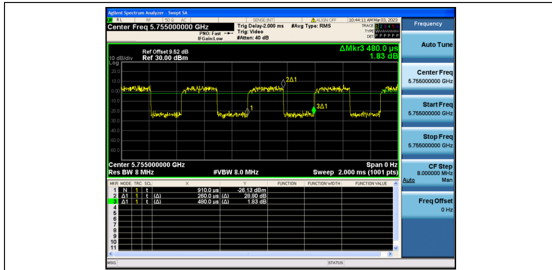
11N40SISO_Ant2_5755
