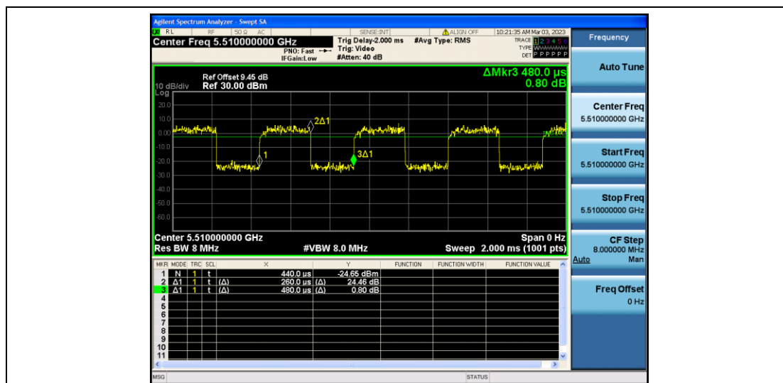
11N40SISO_Ant2_5510
