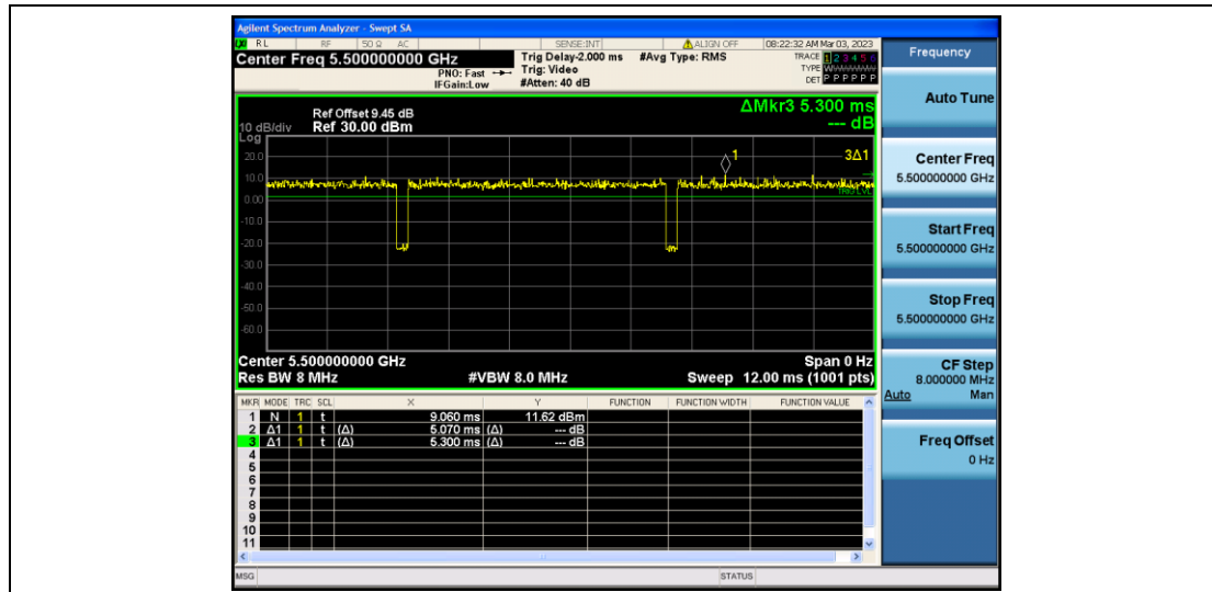
11N20SISO_Ant2_5500
