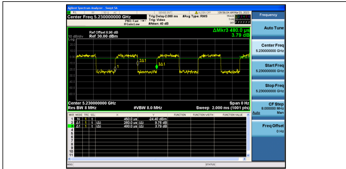
11N40SISO_Ant2_5230
