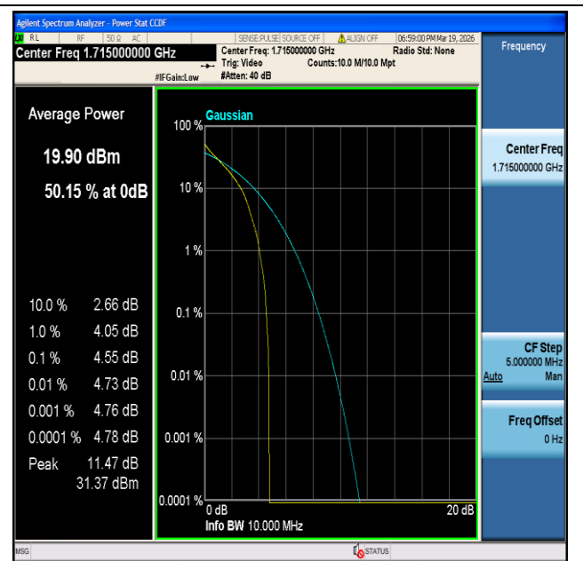
CatM1 Band4-10MHz-QPSK-20000-6#0-PASS
