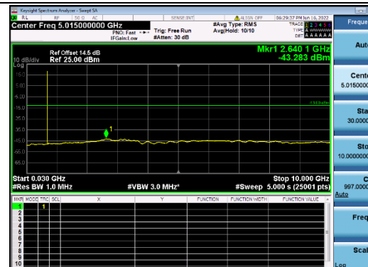
B12-1.4M-Low CH-CSE-1-Q16-1 RB 0
