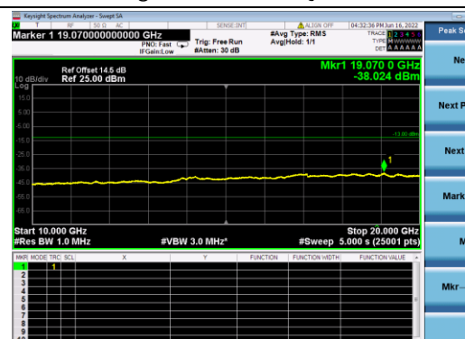
B4-20M-Low CH-CSE-1-Q16-1 RB 0
