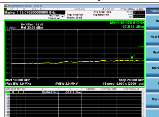
B4-3M-Mid CH-CSE-2-Q16-1 RB 0
