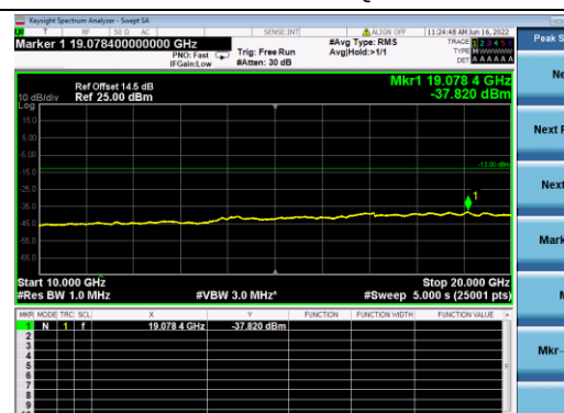
B4-10M-Mid CH-CSE-2-Q16-1 RB 0
