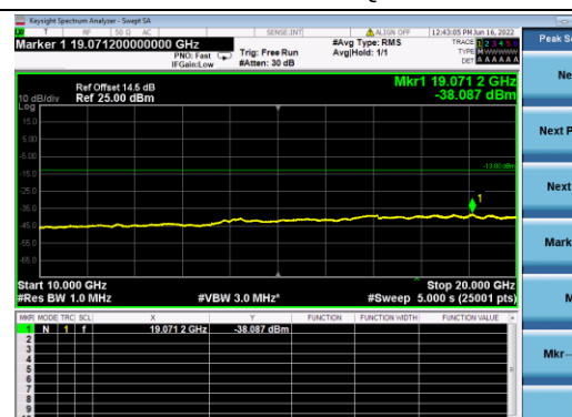
B4-15M-Mid CH-CSE-1-Q16-1 RB 0
