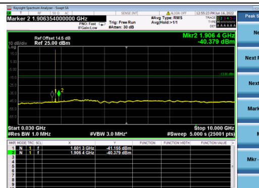
B4-15M-High CH-CSE-2-Q16-1 RB 0
