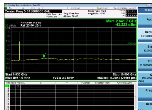
B12-1.4M-Mid CH-CSE-1-Q16-1 RB 0
