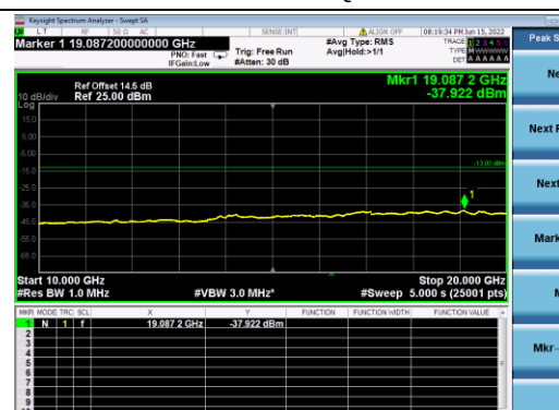
B4-5M-Mid CH-CSE-2-Q16-1 RB 0
