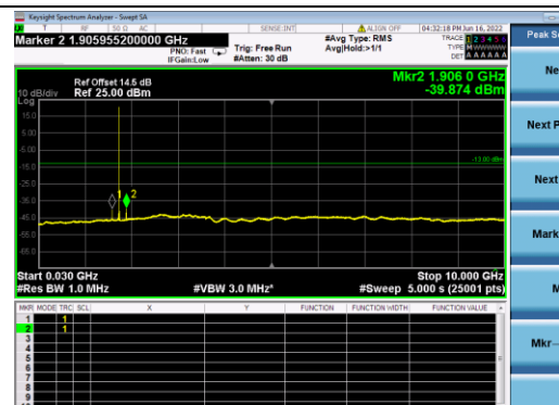
B4-20M-High CH-CSE-2-Q16-1 RB 0
