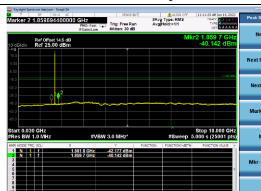
B4-10M-Low CH-CSE-1-Q16-1 RB 0
