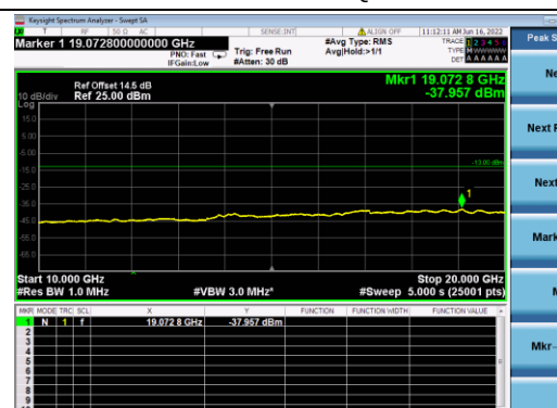
B4-10M-Mid CH-CSE-1-Q16-1 RB 0
