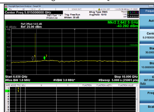
B25-1.4M-High CH-CSE-2-Q16-1 RB 0
