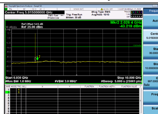
B25-1.4M-Low CH-CSE-2-Q16-1 RB 0
