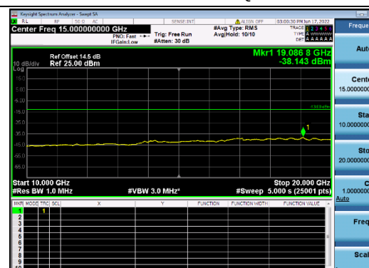
B25-15M-High CH-CSE-1-Q16-1 RB 0
