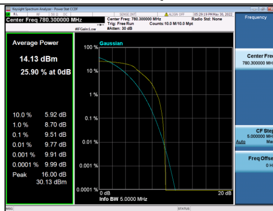
B13-5M-Mid CH-PAPR-QPSK
