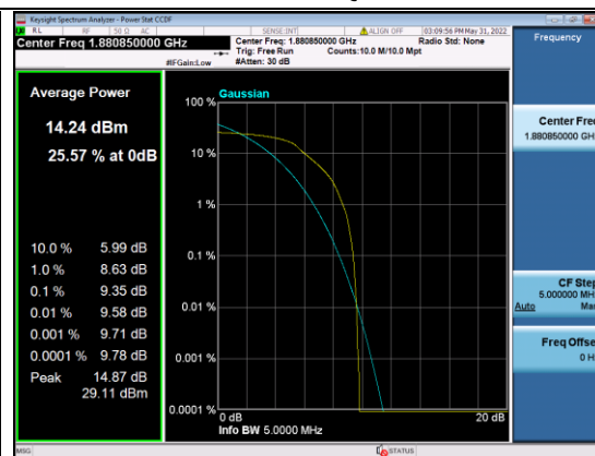
B25-5M-Mid CH-PAPR-QPSK
