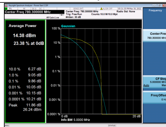
B13-5M-Mid CH-PAPR-Q16
