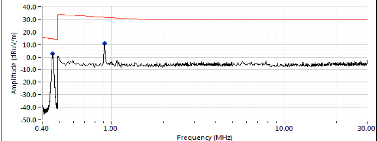
EUT Upright - Close Loop
