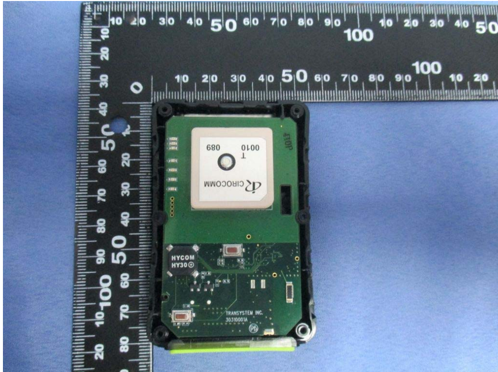
(16) EUT Photo
