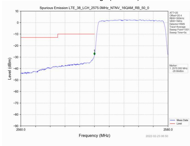
Lower Band Edge (16-QAM)
