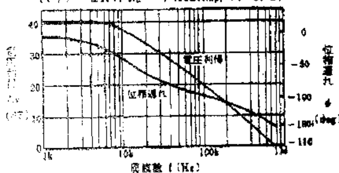
電圧利得, 位相遅れ対周波数特性例
