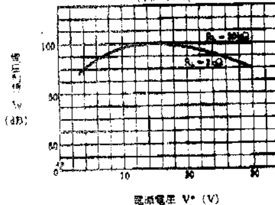
電圧利得対電源電圧特性例
