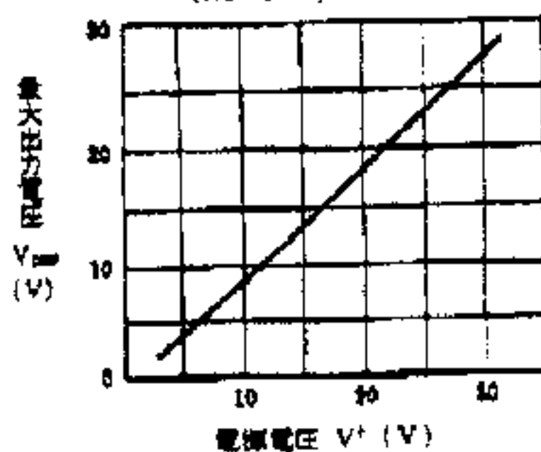
最大出力電圧対電源電圧特性例
