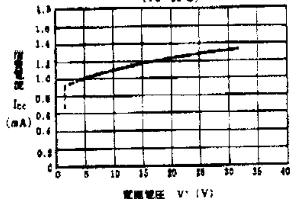
消費電流対電源電圧特性例
