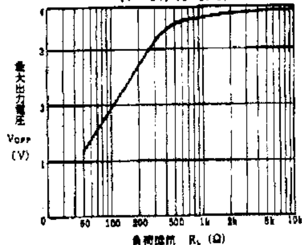
最大出力電圧対負荷特性例
