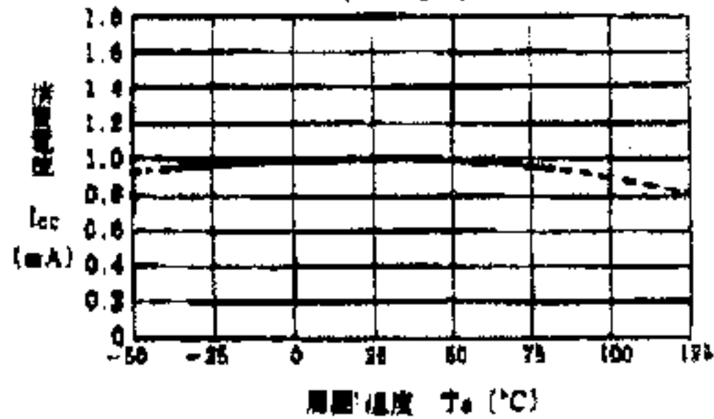
消費電流温度特性例 ( V^+ = 5V )
