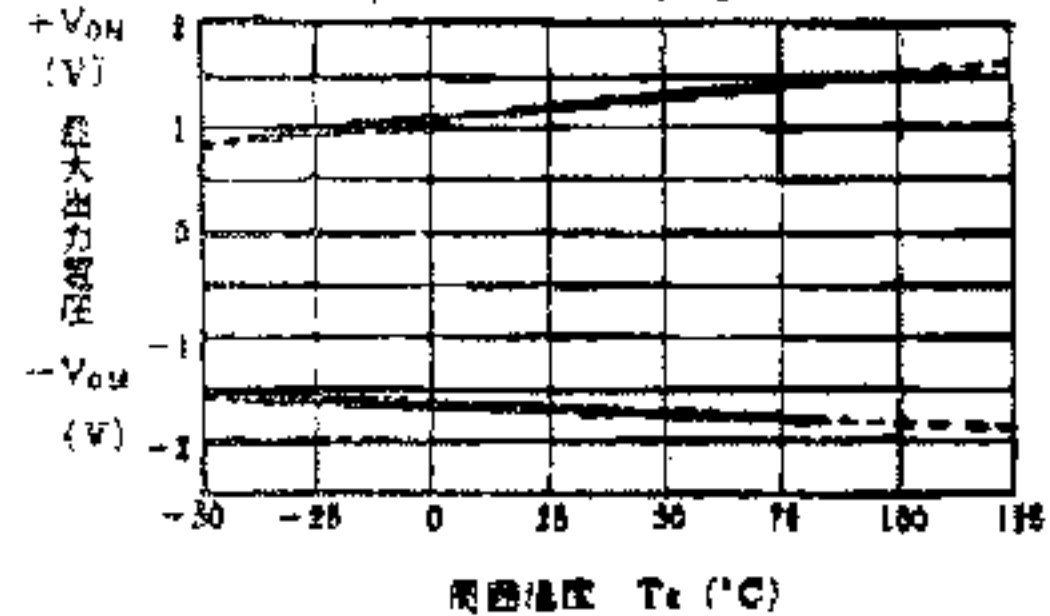
最大出力電圧温度特性例 ( V^+/V^- = \pm 2.5V, R_L = 1k\Omega )
