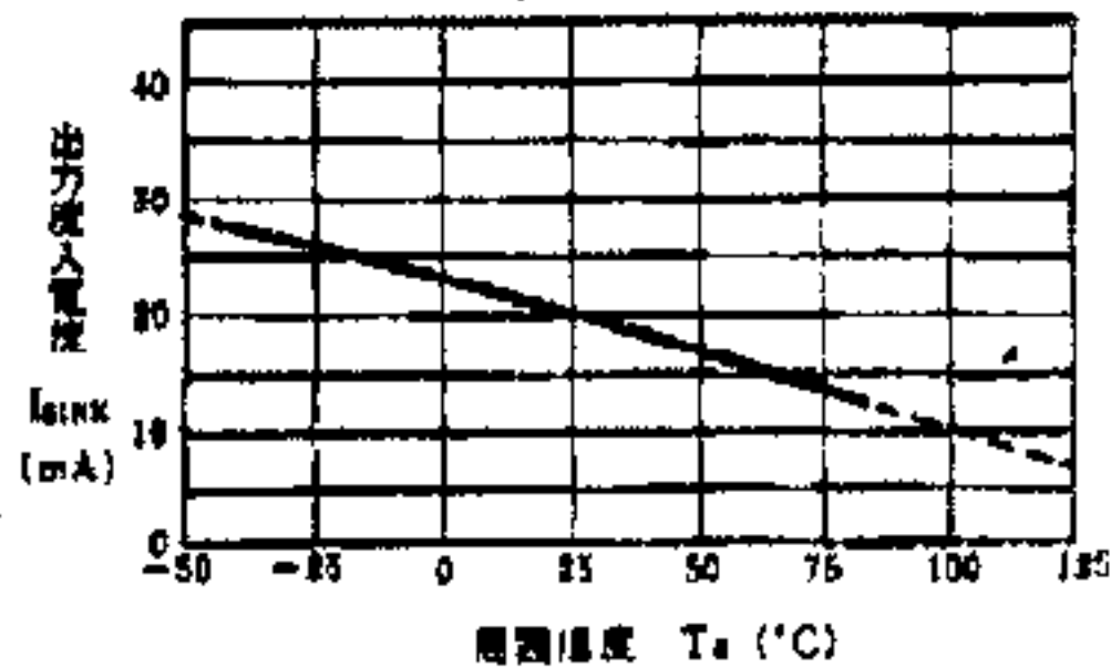
出力流入電流温度特性例 ( V^+ = 5V )
