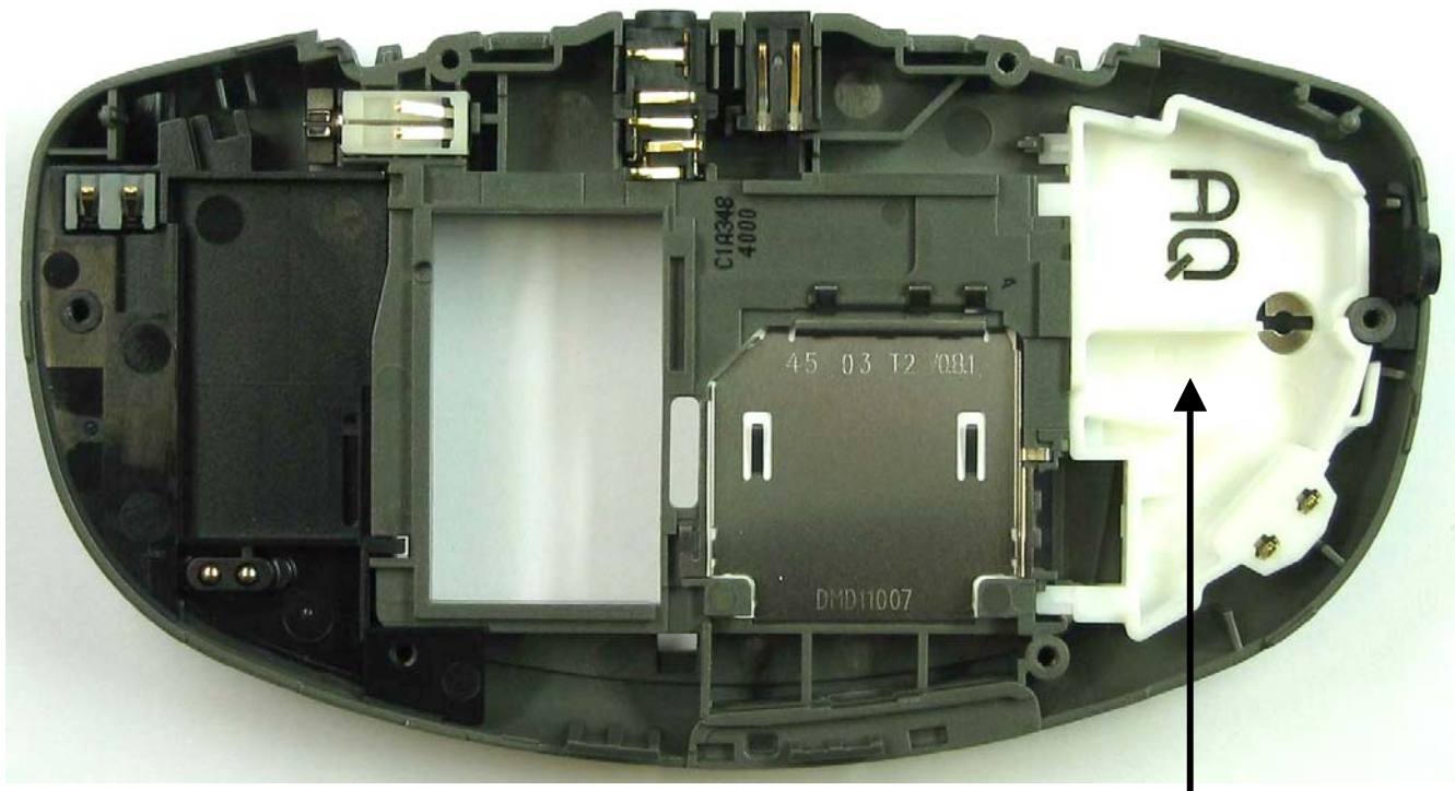
Antenna
