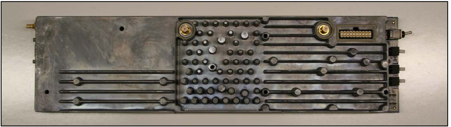
LN Module Right Side
