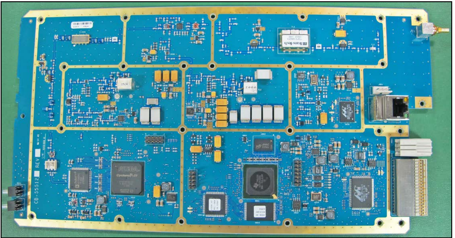
TX Module Bottom
