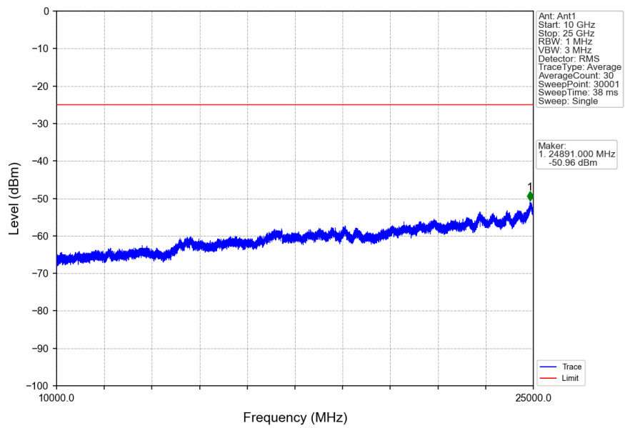
Band7_20MHz_16QAM_MCH_2535MHz_RB_1_0_NTNV
