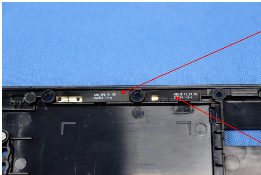
GPS(RX) antenna
