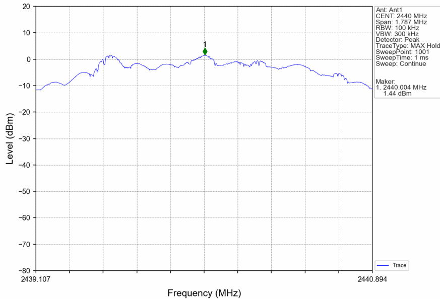
2M_MCH_2440MHz_Ant1_NTNV
