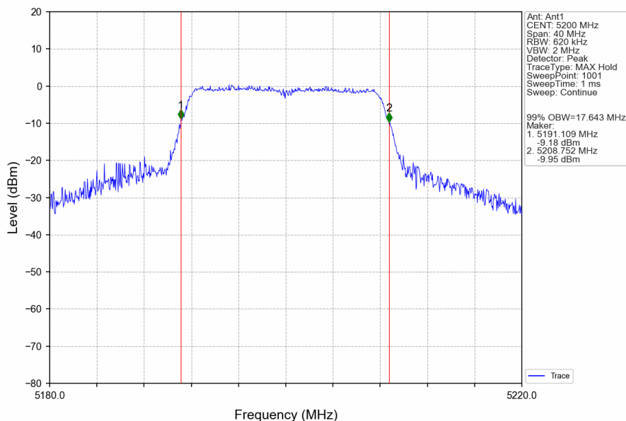
802.11a_MCH_5200MHz_Ant1_NTNV
