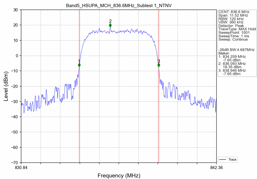
Band5_HSUPA_MCH_836.6MHz_Subtest 1_NTNV
