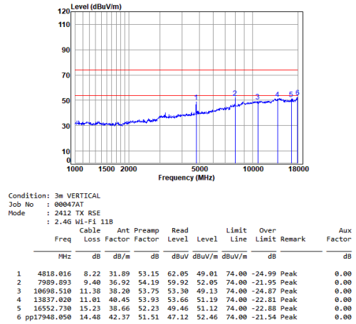
11b_TX_CH_01_Vertical
