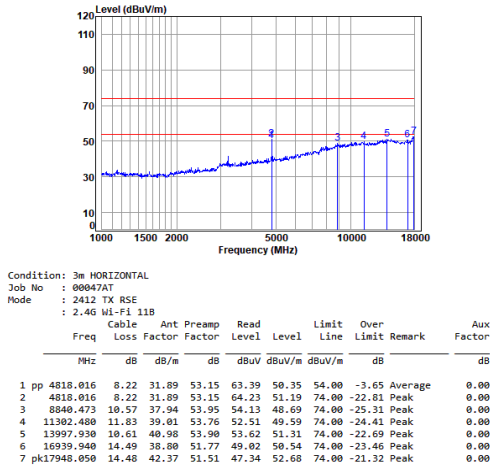
11b_TX_CH_01_Horizontal
