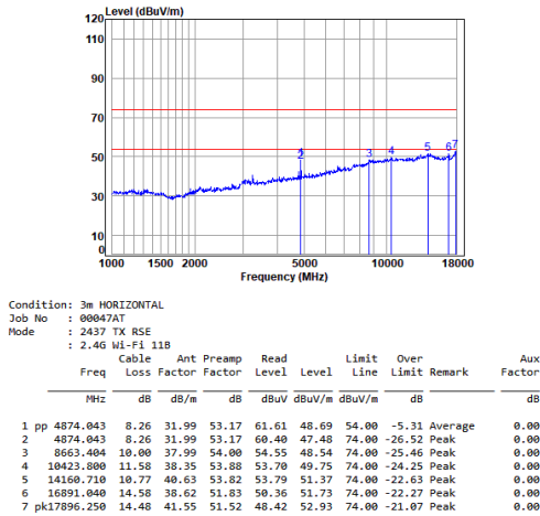
11b_TX_CH_06_Horizontal
