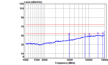
11b_TX_CH_11_Horizontal
