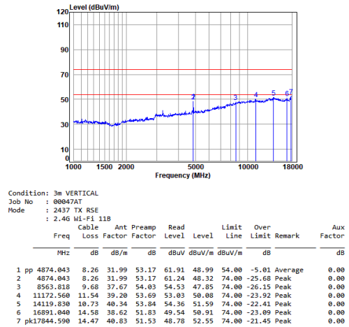
11b_TX_CH_06_Vertical
