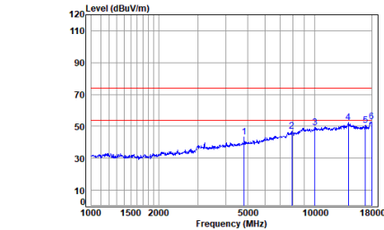
11g_TX_CH_01_Horizontal
