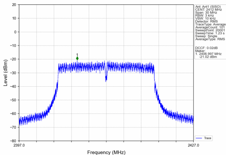
802.11g_LCH_2412MHz_Ant1 (SISO)_NTNV
