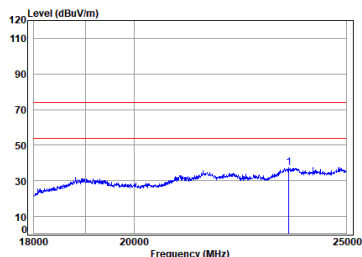
11b_TX_CH_01_Horizontal
