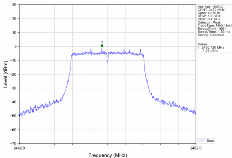
802.11g_HCH_2462MHz_Ant1 (SISO)_NTNV
