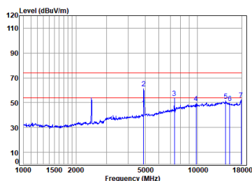
11n_20M_TX_CH_11_Vertical
