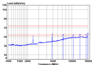
11n_20M_TX_CH_06_Horizontal
