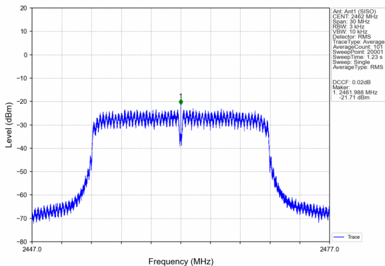
802.11n(HT20)_HCH_2462MHz_Ant1 (SISO)_NTNV
