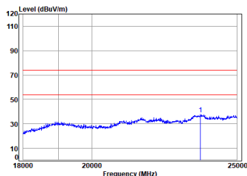
11b_TX_CH_01_Vertical
