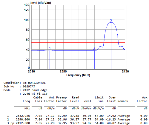
11b_TX_CH_01_Horizontal-Avg
