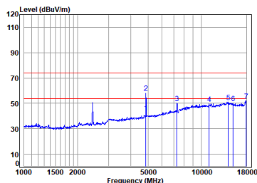
11n_20M_TX_CH_06_Vertical
