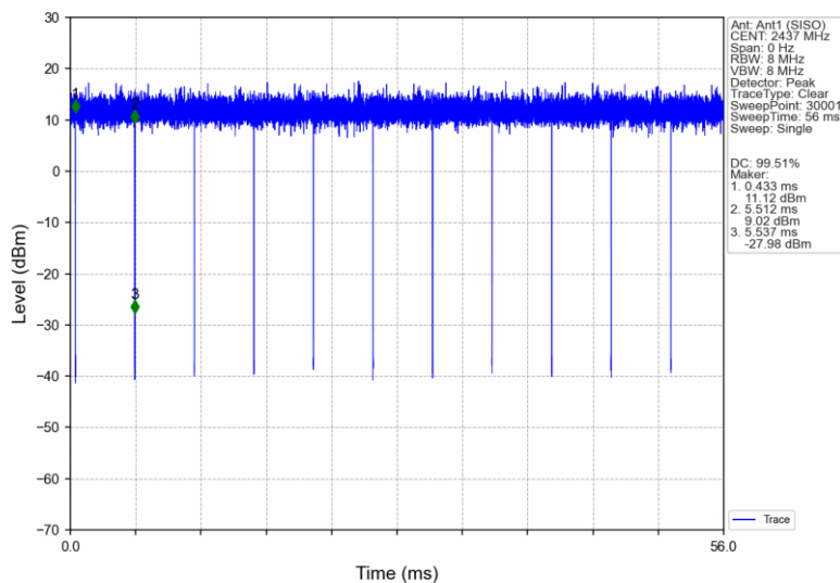
802.11n(HT20)_MCH_2437MHz_Ant1 (SISO)_NTNV
