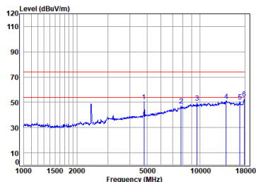
11n_20M_TX_CH_01_Horizontal
