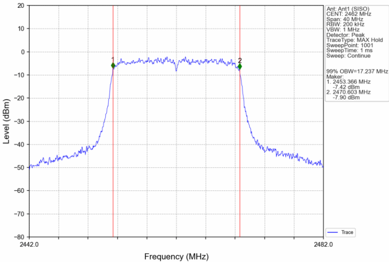
802.11n(HT20)_HCH_2462MHz_Ant1 (SISO)_NTNV
