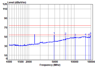
11g_TX_CH_11_Horizontal
