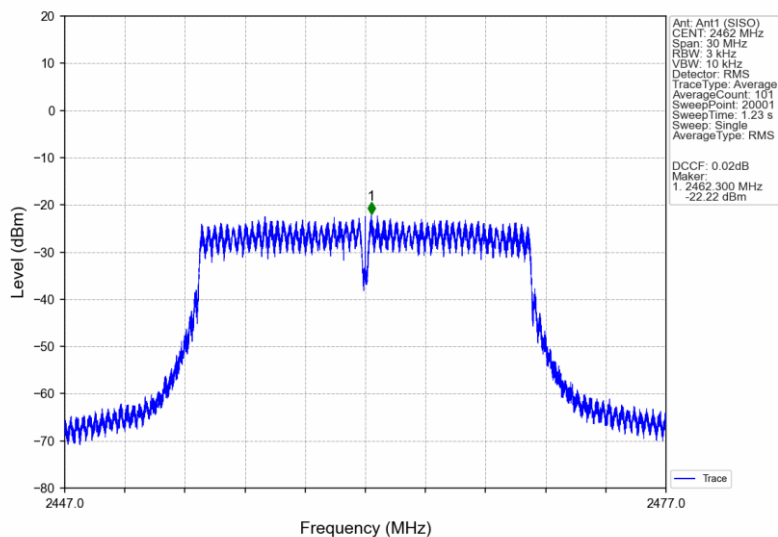
802.11g_HCH_2462MHz_Ant1 (SISO)_NTNV
