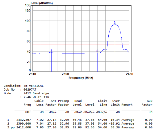
11b_TX_CH_01_Vertical-Avg
