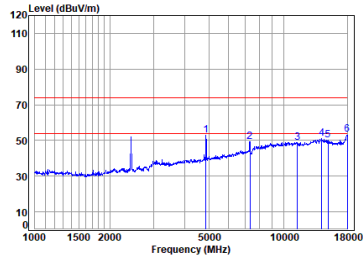
11g_TX_CH_06_Horizontal
