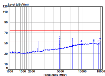
11n_20M_TX_CH_11_Horizontal
