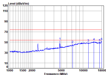
11n_20M_TX_CH_01_Vertical
