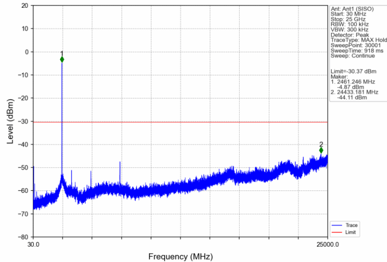
802.11n(HT20)_HCH_2462MHz_Ant1 (SISO)_NTNV
