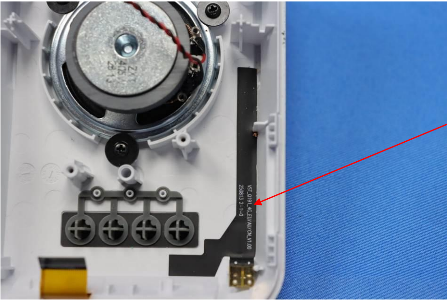
WWAN antenna
