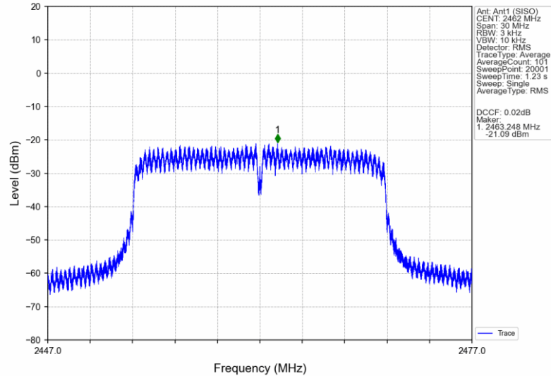
802.11n(HT20)_HCH_2462MHz_Ant1 (SISO)_NTNV
