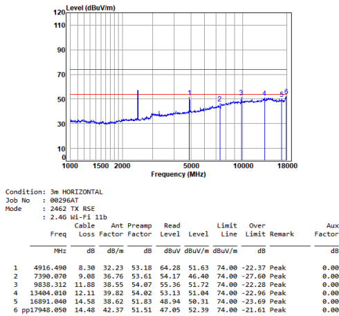
11b_TX_CH_11_Horizontal
