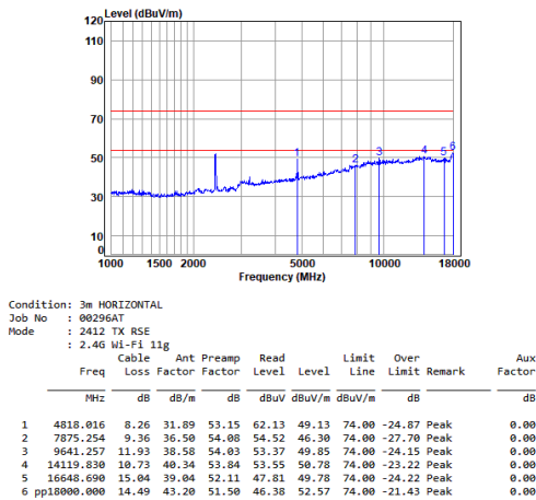
11g_TX_CH_01_Horizontal
