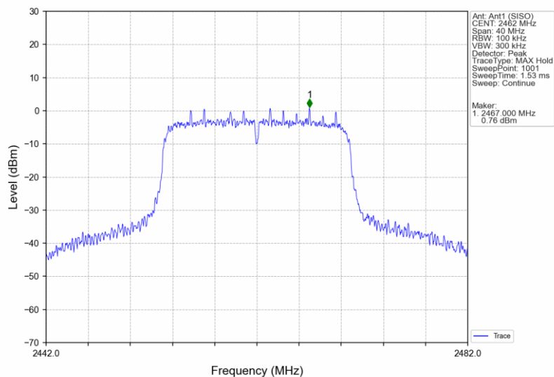
802.11n(HT20)_HCH_2462MHz_Ant1 (SISO)_NTNV
