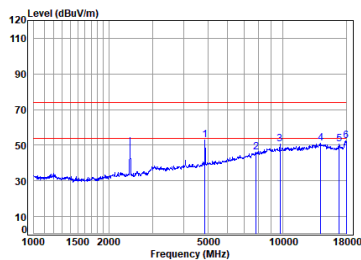
11b_TX_CH_06_Vertical
