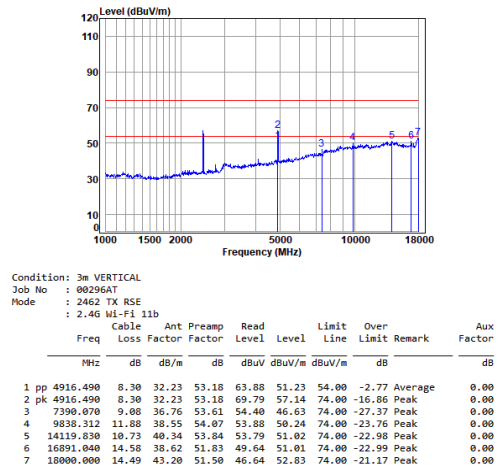
11b_TX_CH_11_Vertical
