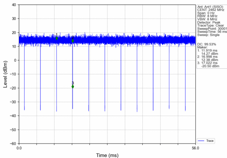
802.11n(HT20)_HCH_2462MHz_Ant1 (SISO)_NTNV
