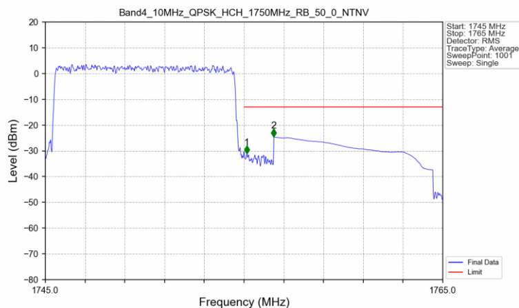
Band4_10MHz_QPSK_HCH_1750MHz_RB_50_0_NTNV
