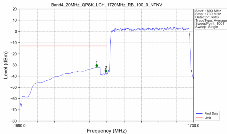
Band4_20MHz_QPSK_LCH_1720MHz_RB_100_0_NTNV
