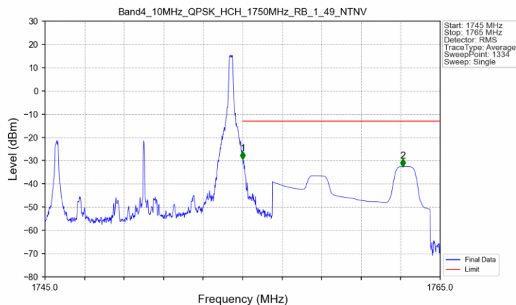
Band4_10MHz_QPSK_HCH_1750MHz_RB_1_49_NTNV
