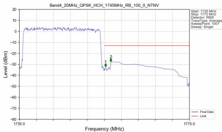
Band4_20MHz_QPSK_HCH_1745MHz_RB_100_0_NTNV
