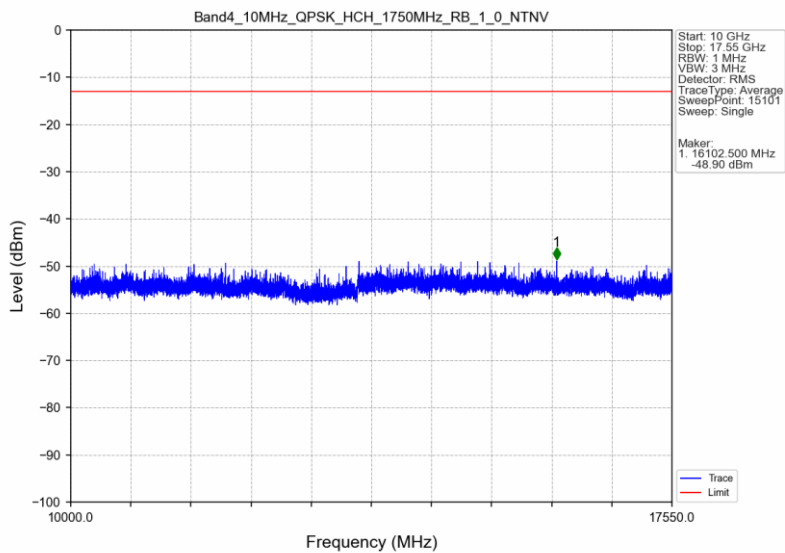
Band4_10MHz_QPSK_HCH_1750MHz_RB_1_0_NTNV
