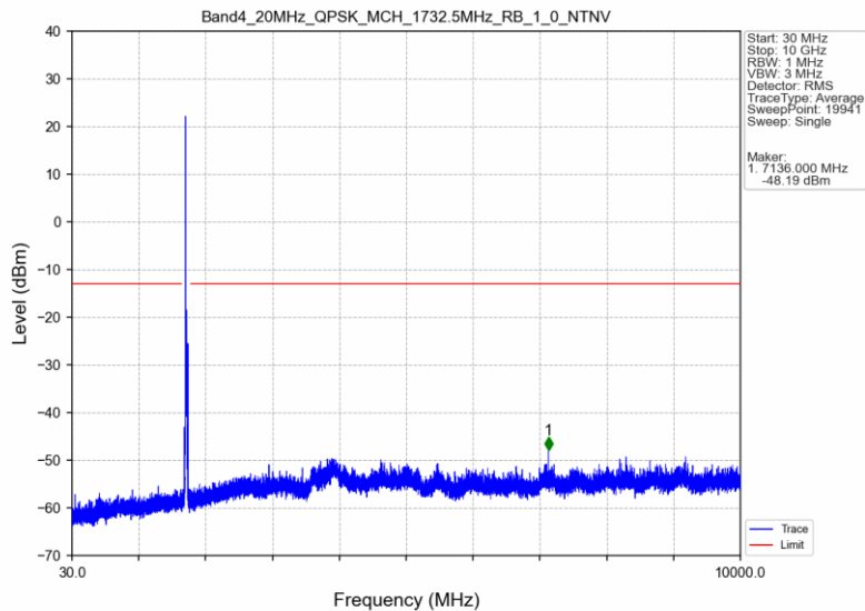
Band4_20MHz_QPSK_MCH_1732.5MHz_RB_1_0_NTNV
