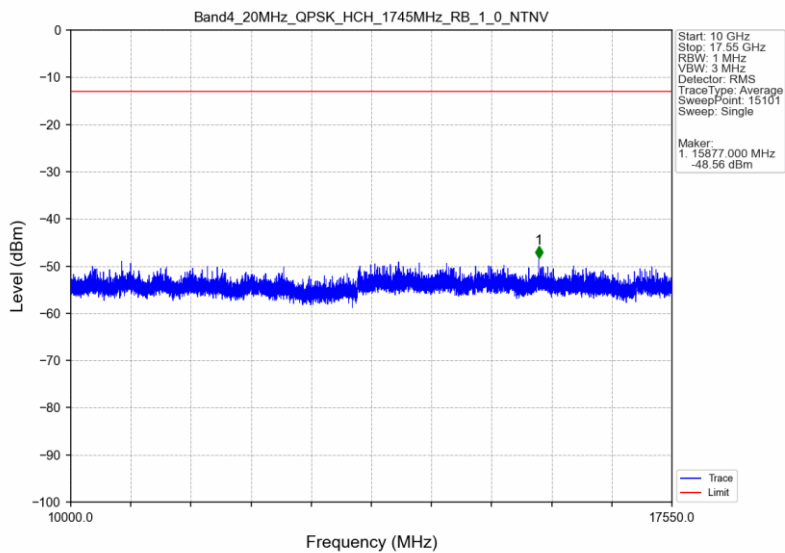
Band4_20MHz_QPSK_HCH_1745MHz_RB_1_0_NTNV
