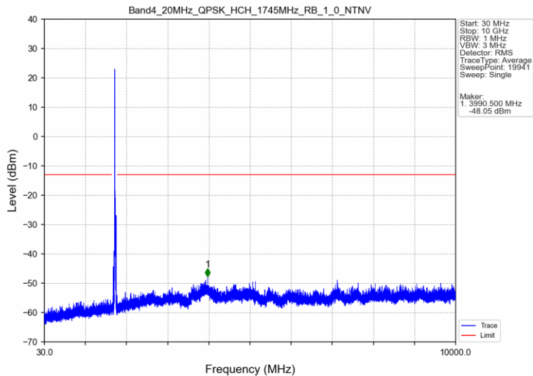
Band4_20MHz_QPSK_HCH_1745MHz_RB_1_0_NTNV
