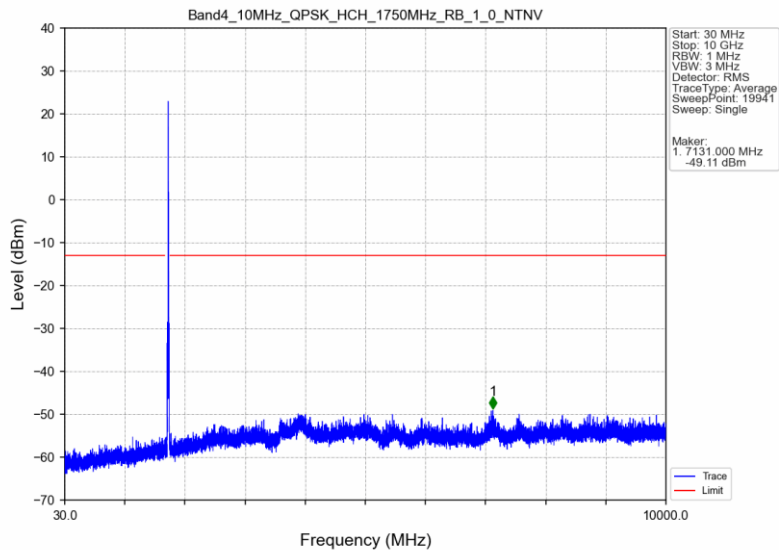
Band4_10MHz_QPSK_HCH_1750MHz_RB_1_0_NTNV
