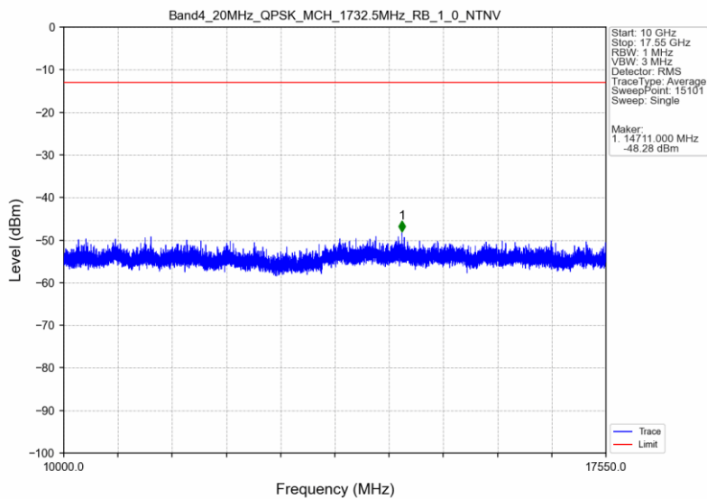
Band4_20MHz_QPSK_MCH_1732.5MHz_RB_1_0_NTNV
