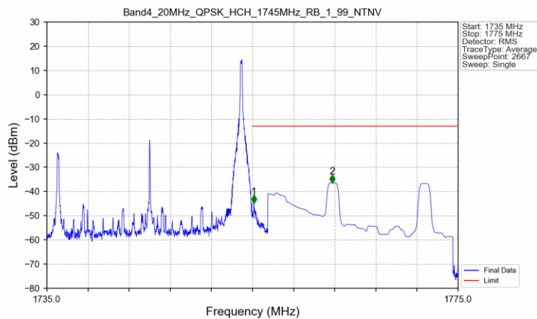
Band4_20MHz_QPSK_HCH_1745MHz_RB_1_99_NTNV
