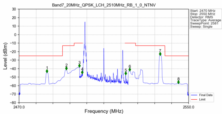
Band7_20MHz_QPSK_LCH_2510MHz_RB_1_0_NTNV
