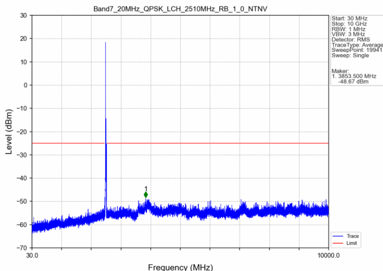
Band7_20MHz_QPSK_LCH_2510MHz_RB_1_0_NTNV
