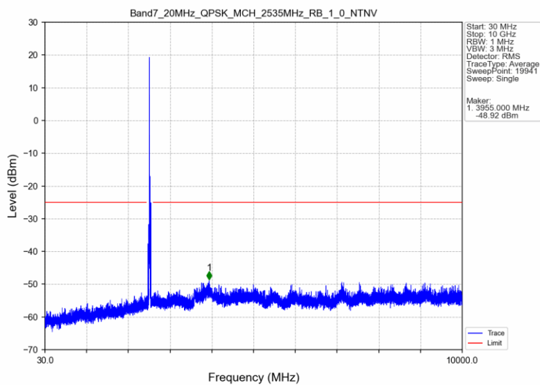
Band7_20MHz_QPSK_MCH_2535MHz_RB_1_0_NTNV
