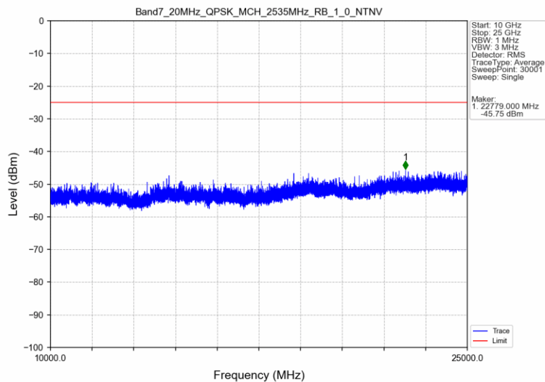
Band7_20MHz_QPSK_MCH_2535MHz_RB_1_0_NTNV
