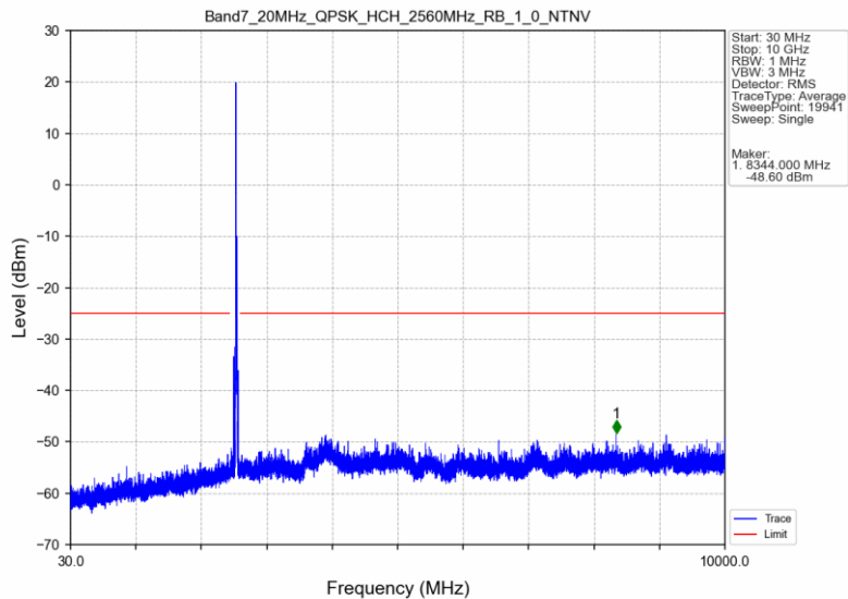
Band7_20MHz_QPSK_HCH_2560MHz_RB_1_0_NTNV
