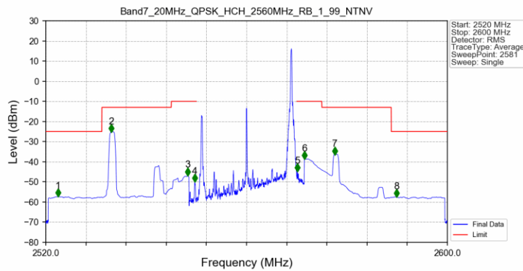
Band7_20MHz_QPSK_HCH_2560MHz_RB_1_99_NTNV
