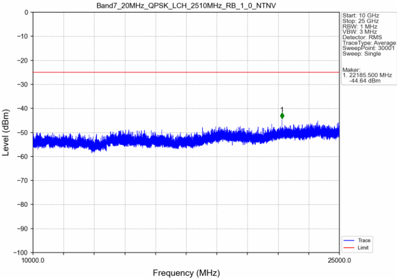
Band7_20MHz_QPSK_LCH_2510MHz_RB_1_0_NTNV
