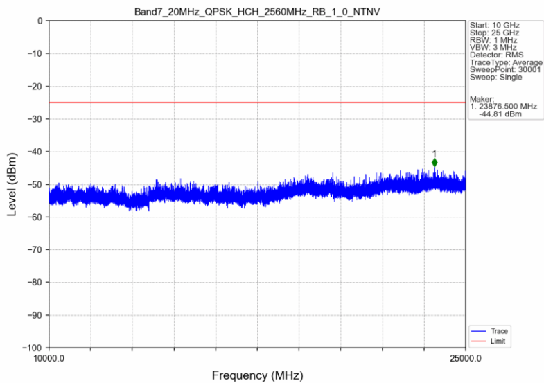
Band7_20MHz_QPSK_HCH_2560MHz_RB_1_0_NTNV
