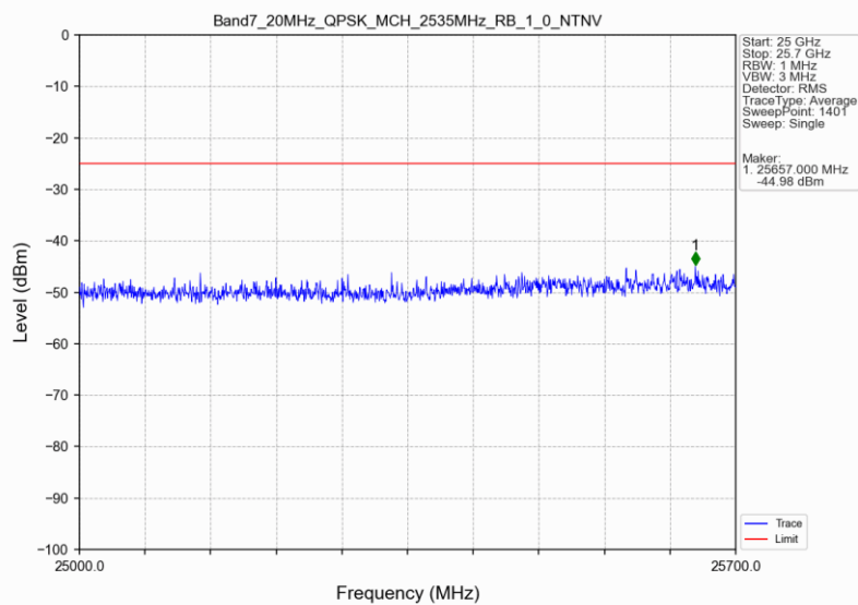
Band7_20MHz_QPSK_MCH_2535MHz_RB_1_0_NTNV
