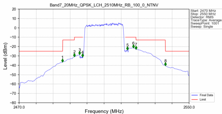
Band7_20MHz_QPSK_LCH_2510MHz_RB_100_0_NTNV
