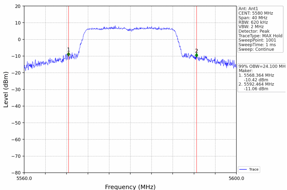
802.11n(HT20)_MCH_5580MHz_Ant1_NTNV
