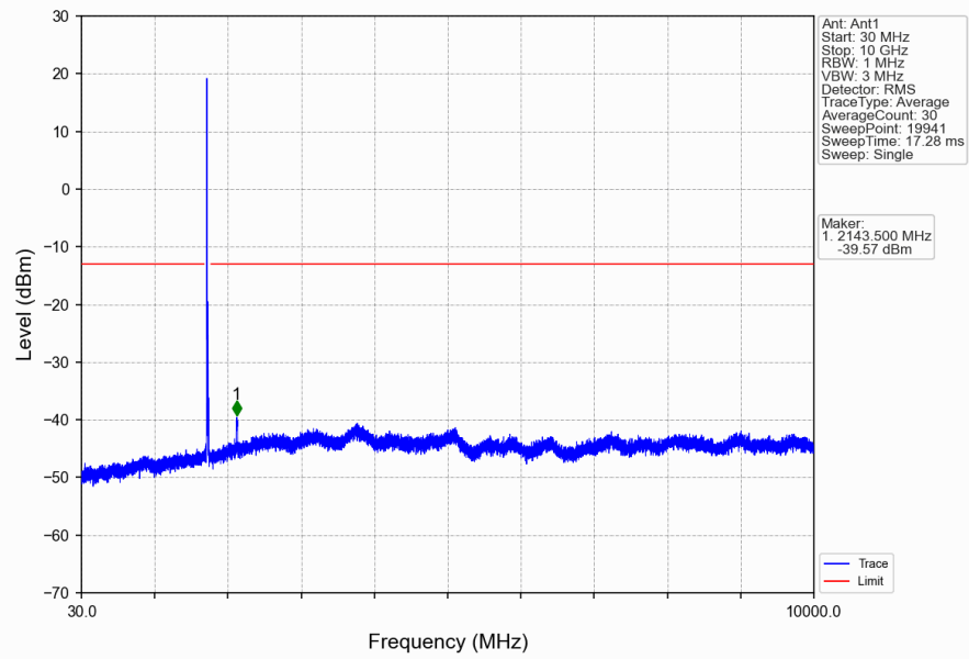
Band4_20MHz_QPSK_HCH_1745MHz_RB_1_0_NTNV
