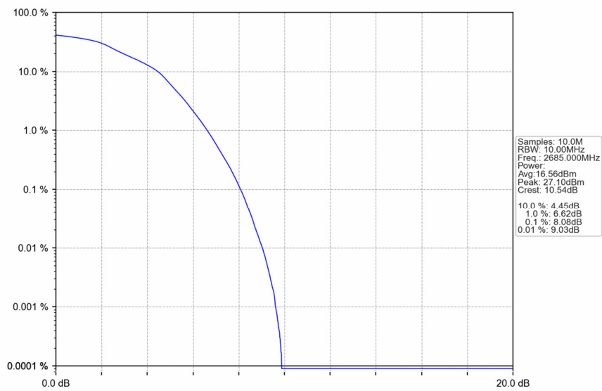
Band41 10MHz 16QAM HCH 2685MHz RB 50 0 NTNV
