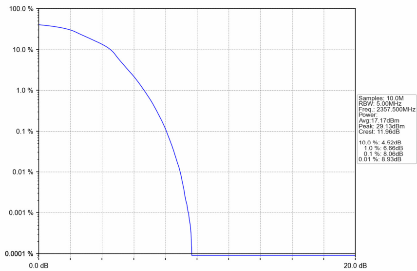
Band40b 5MHz 16QAM HCH 2357.5MHz RB 25 0 NTNV
