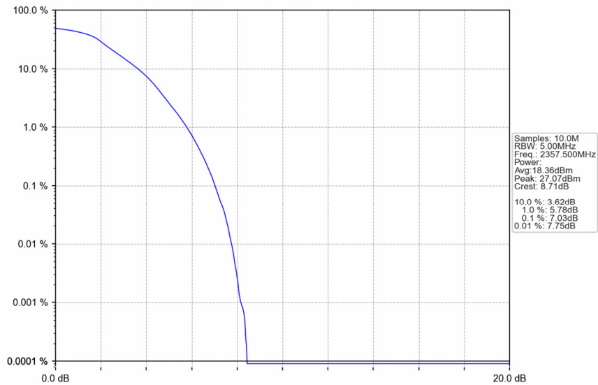
Band40b 5MHz QPSK HCH 2357.5MHz RB 25 0 NTNV
