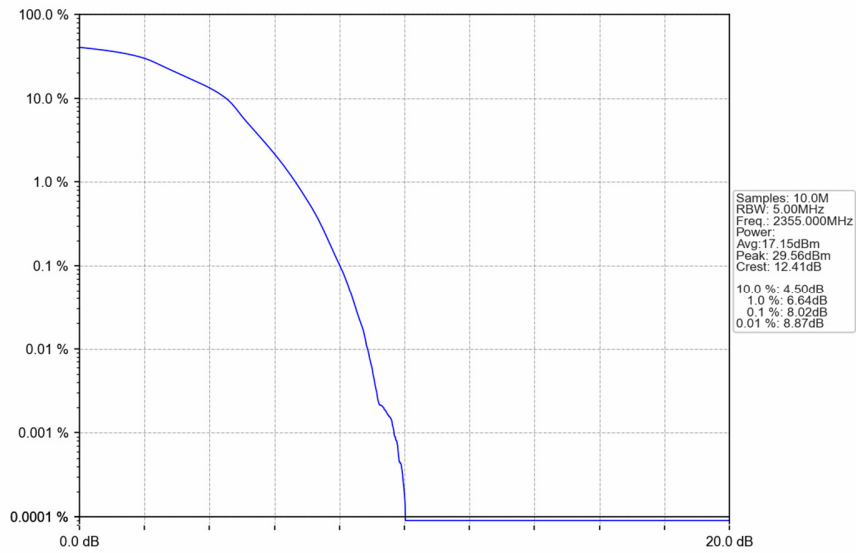
Band40b 5MHz 16QAM MCH 2355MHz RB 25 0 NTNV
