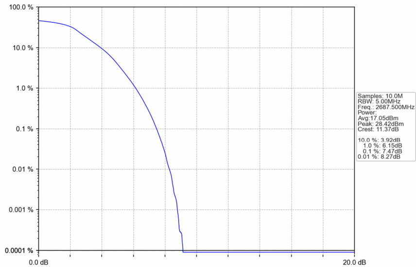
Band41 5MHz QPSK HCH 2687.5MHz RB 25 0 NTNV
