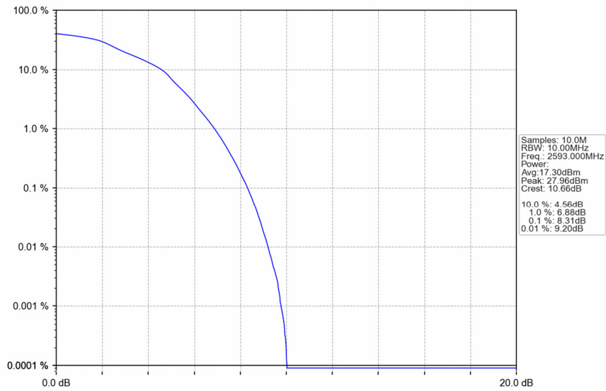
Band41 10MHz 16QAM MCH 2593MHz RB 50 0 NTNV
