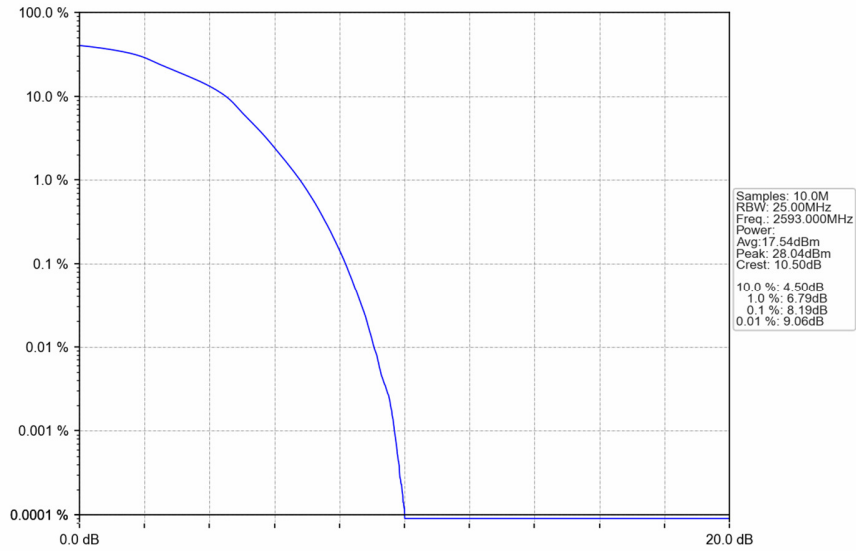
Band41 20MHz 16QAM MCH 2593MHz RB 100 0 NTN
