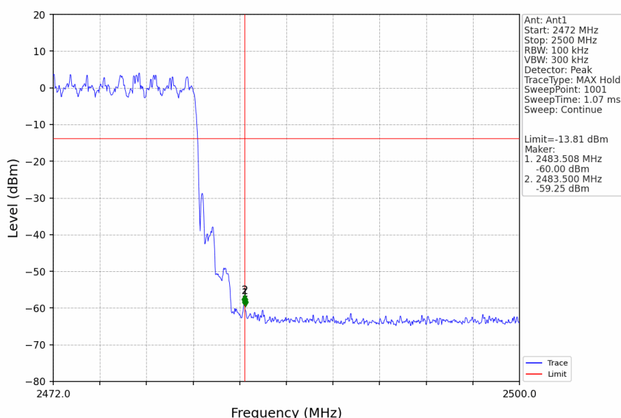
Pi/4DQPSK_2DH5_HOPP_Ant1_NTNV
