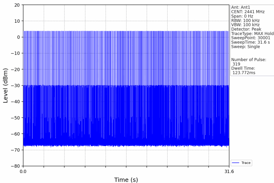
Pi/4DQPSK_2DH1_HOPP_Ant1_NTNV
