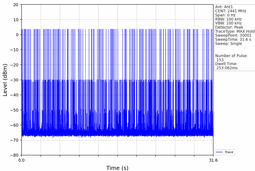
Pi/4DQPSK_2DH3_HOPP_Ant1_NTNV
