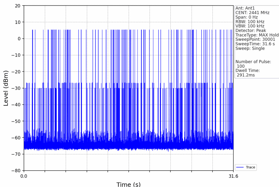
GFSK_DH5_HOPP_Ant1_NTNV
