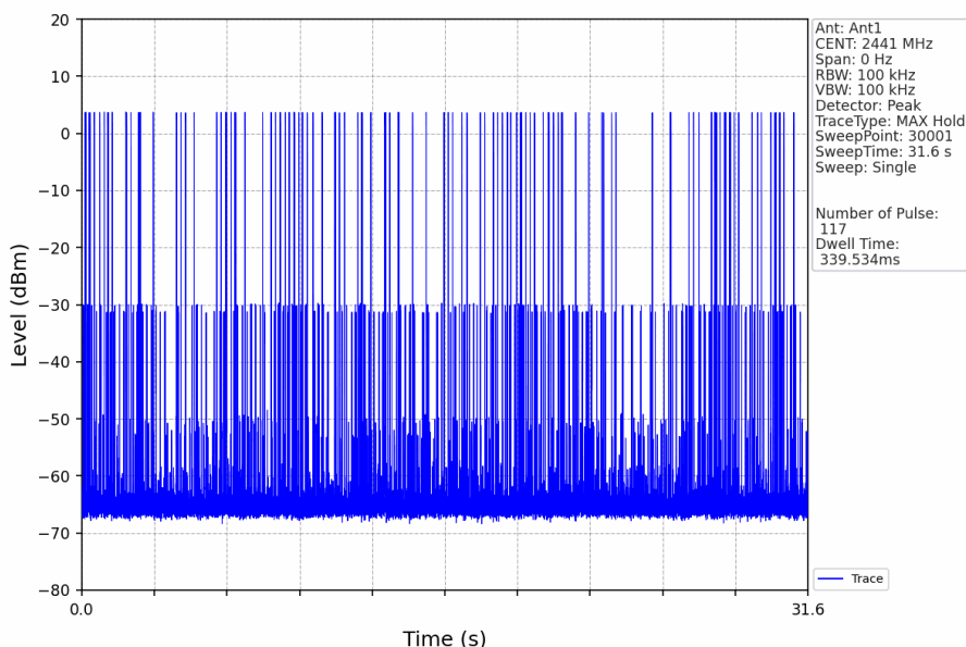
Pi/4DQPSK_2DH5_HOPP_Ant1_NTNV
