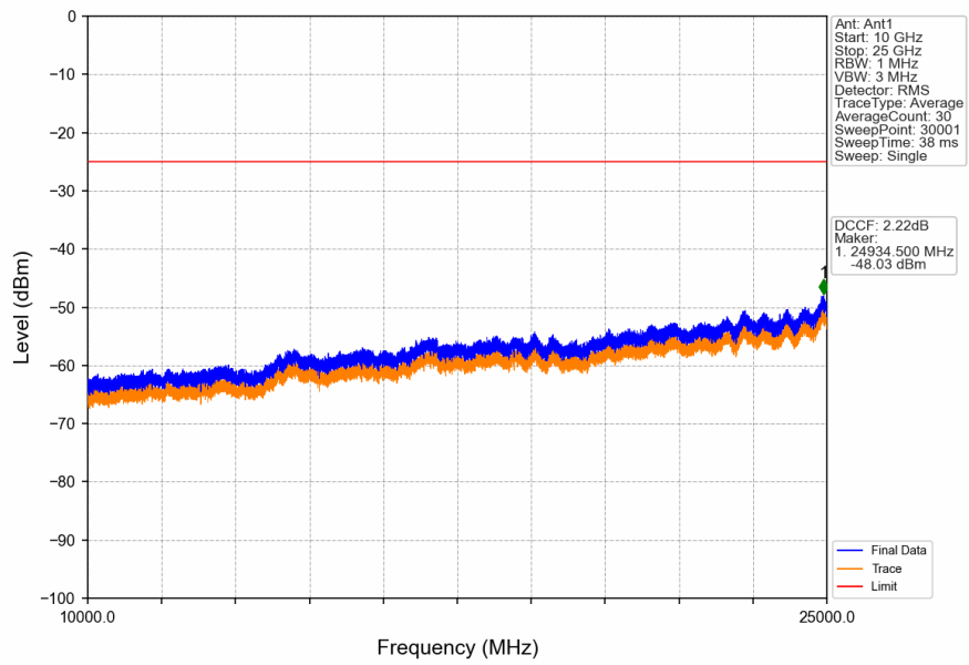
Band38_10MHz_QPSK_LCH_2575MHz_RB_1_0_NTNV
