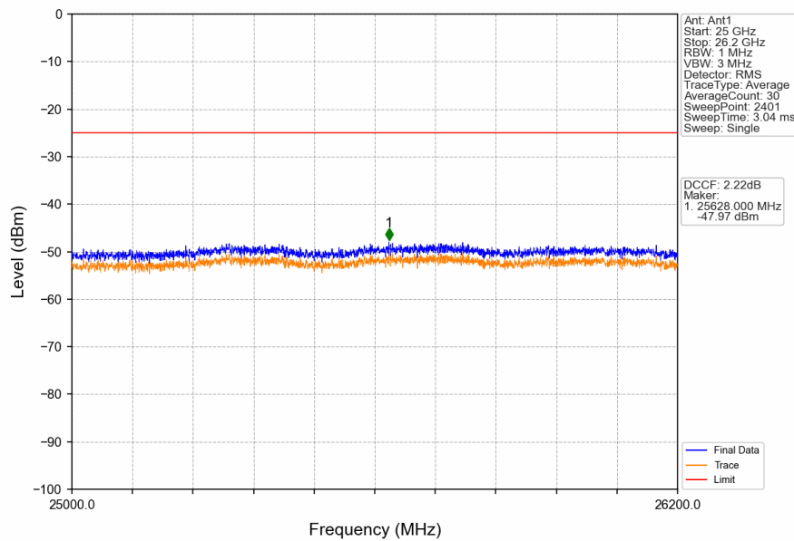
Band38_10MHz_QPSK_LCH_2575MHz_RB_1_0_NTNV
